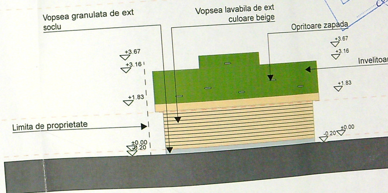
Fatada Sud
