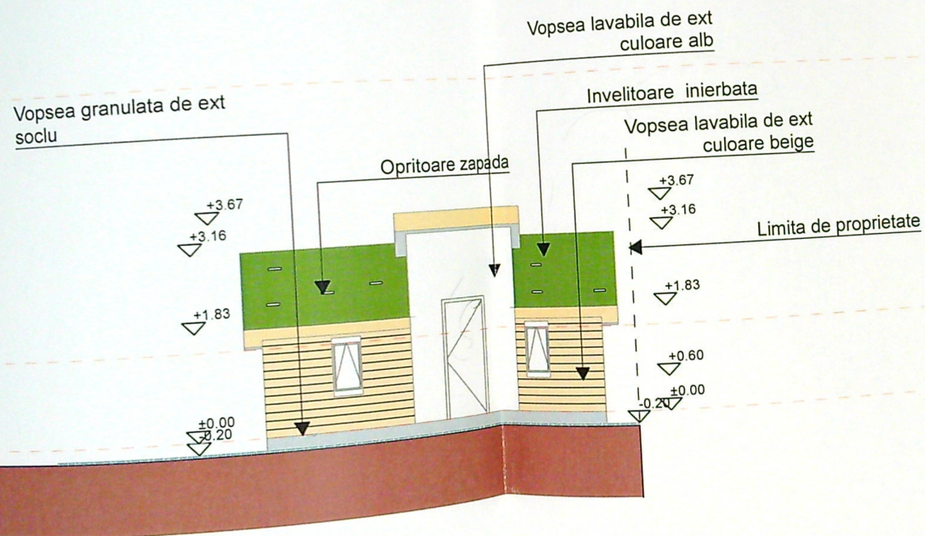
Fatada Nord
