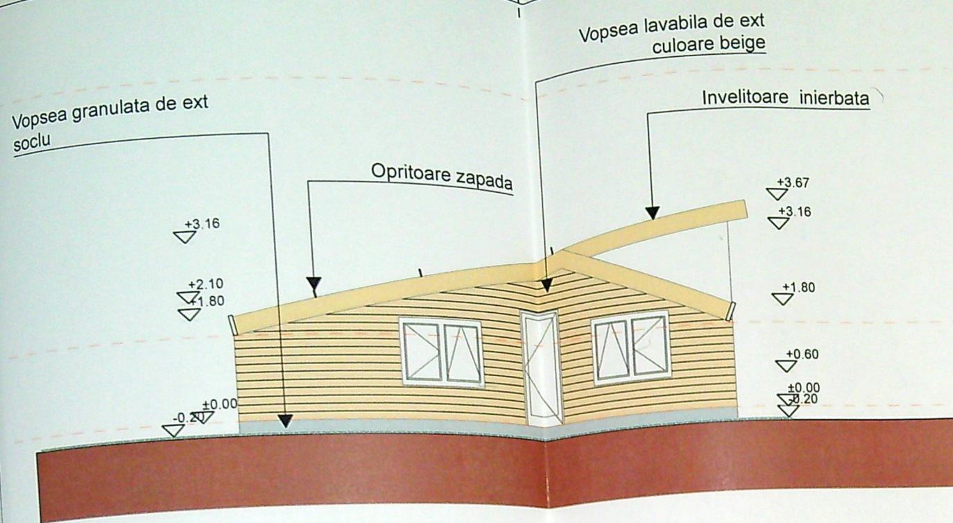
Fatada Est
