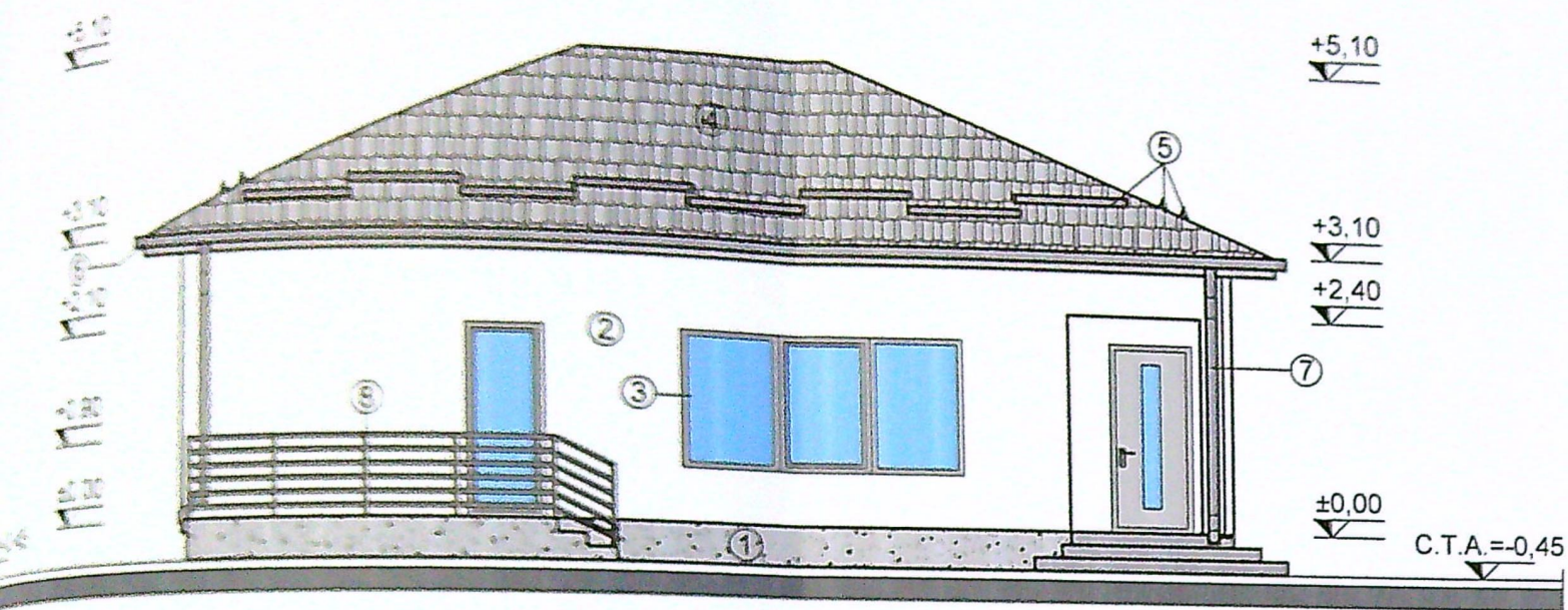
FATADA PRINCIPALA - NORD-VEST
