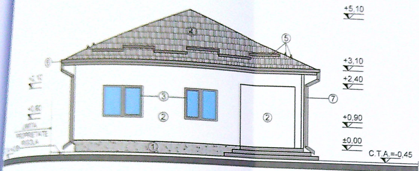
FATADA PRINCIPALA - NORD-VEST
