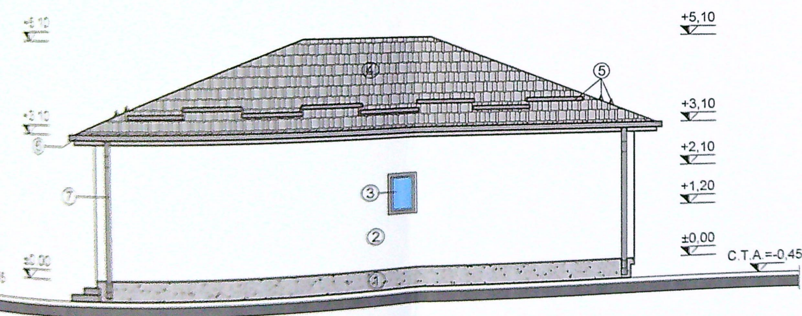
FATADA SECUNDARA - SUD-EST
