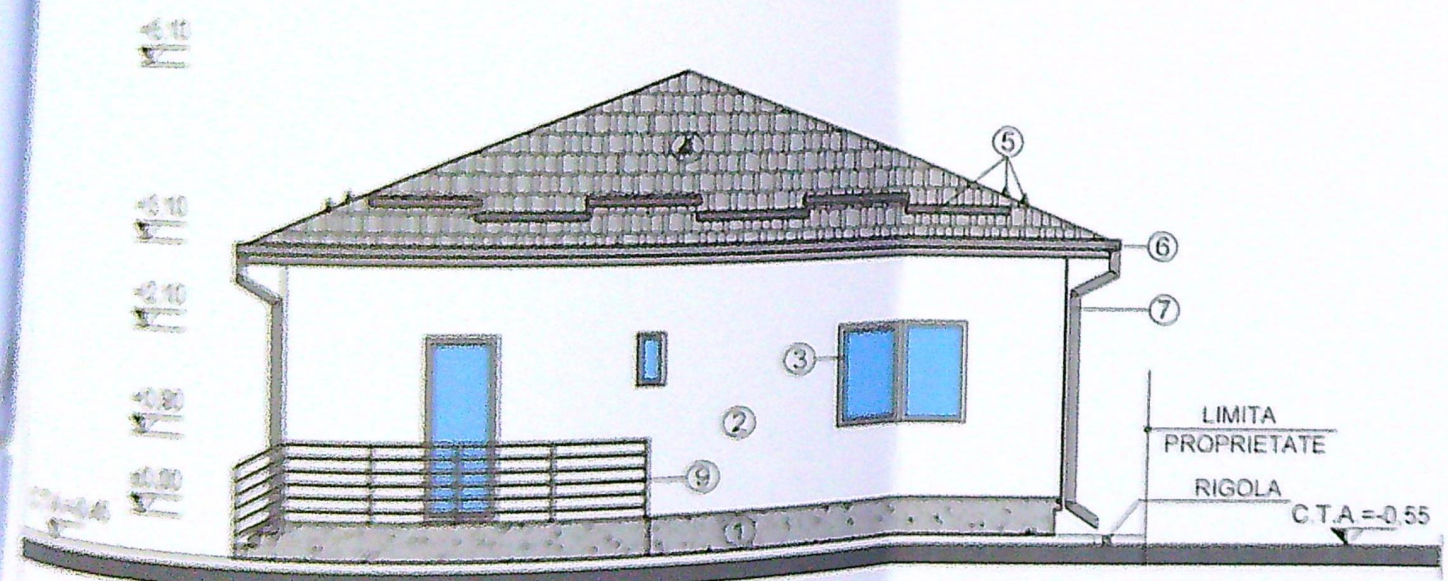
FATADA SECUNDARA - SUD-EST
