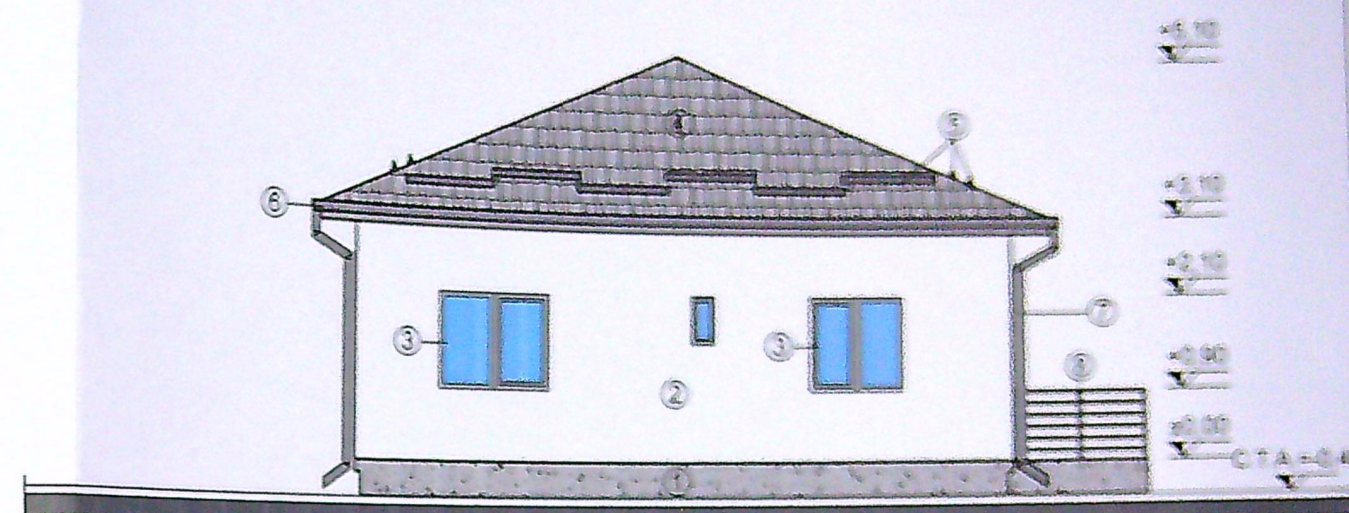
FATADA LATERALA STANGA - NORD-EST
