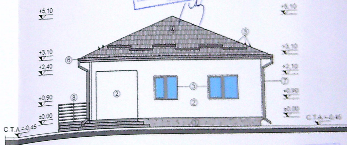
FATADA LATERALA DREAPTA - SUD-VEST
