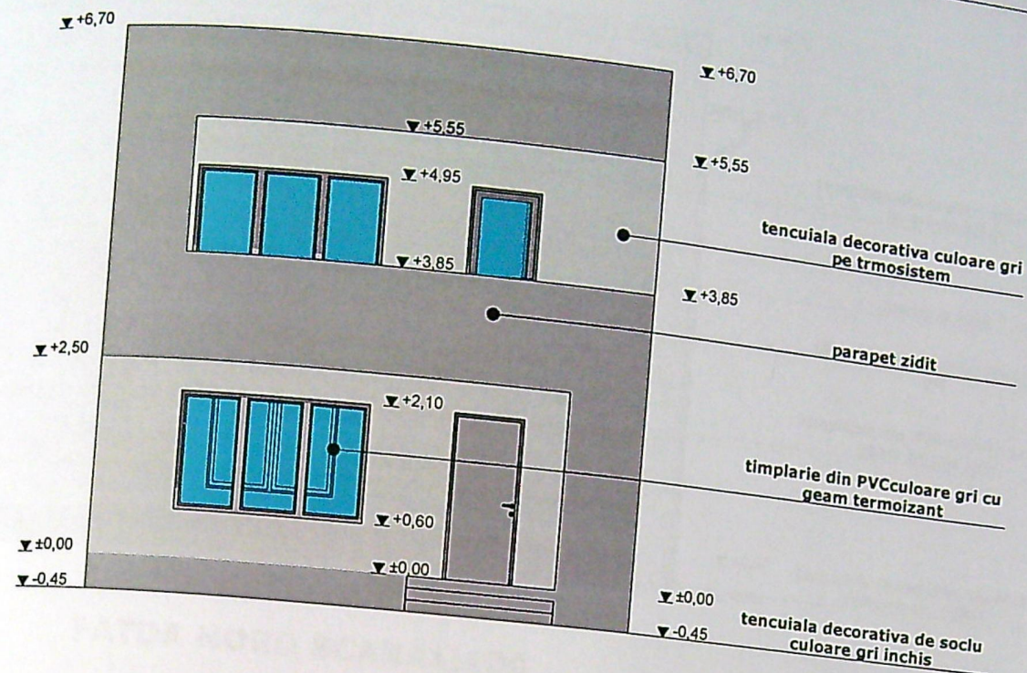
FATADA EST SCARA1:100
