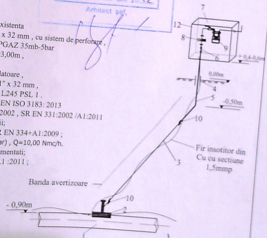
SCHEMA IZOMETRICA RACORD GAZE NATURALE R.P.
