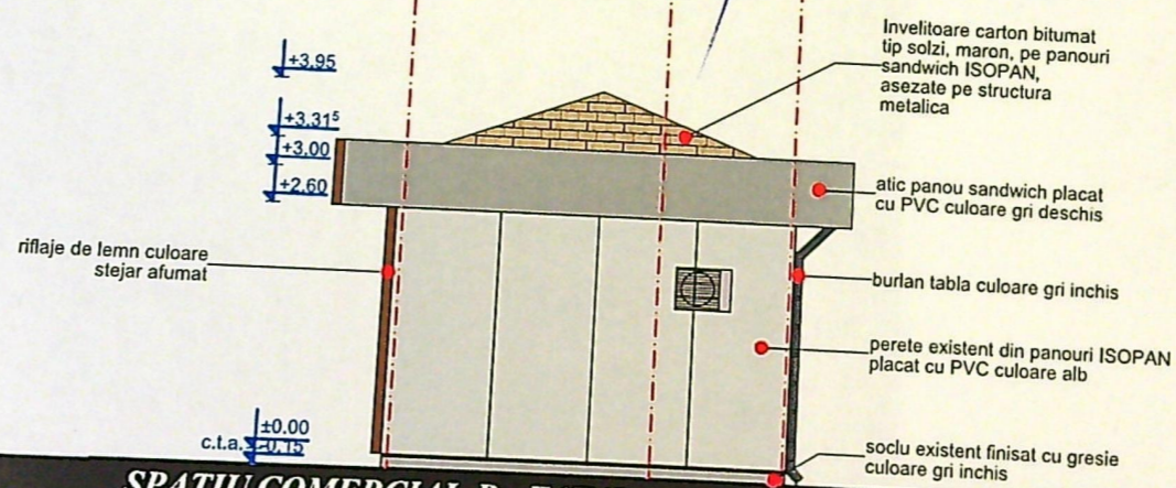
SPATIU COMERCIAL P - FATADA VEST - SITUATIE PROPUSA
