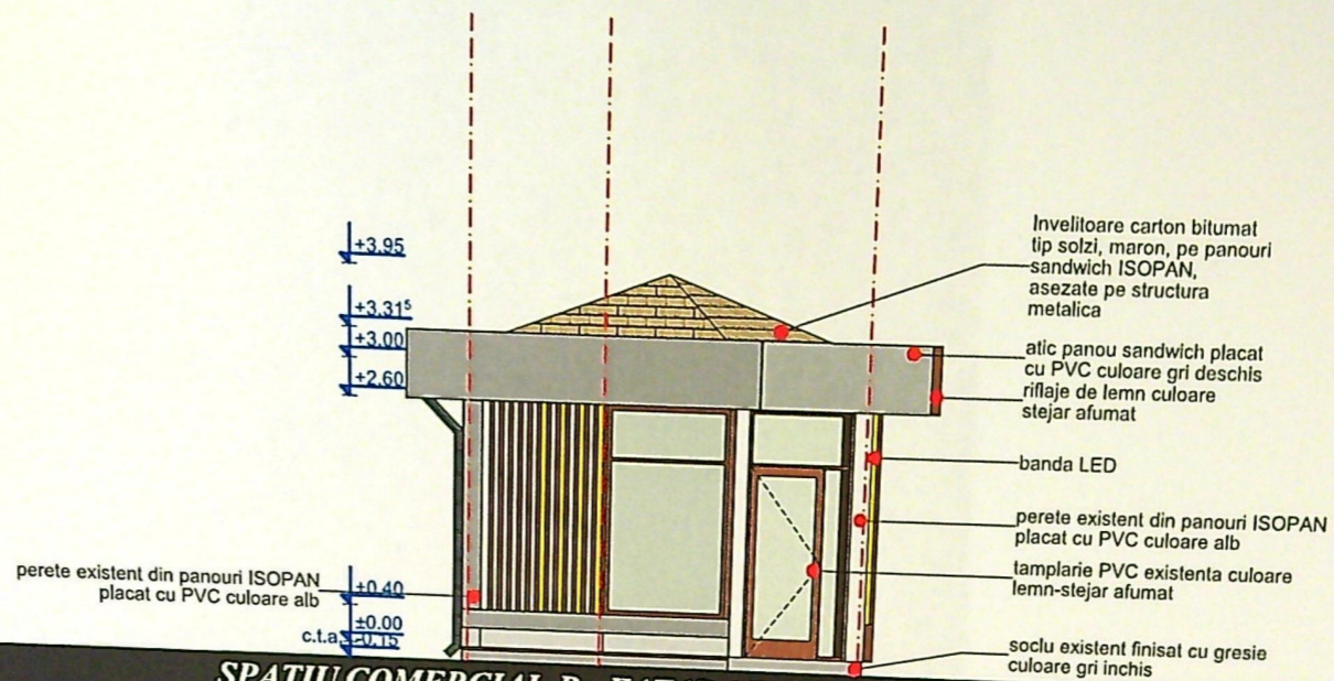
SPATIU COMERCIAL P - FATADA EST - SITUATIE PROPUSA
