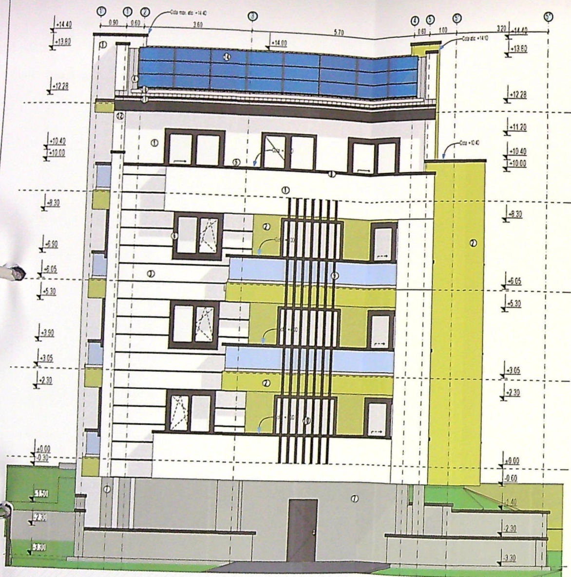
FATADA POSTERIOARA
