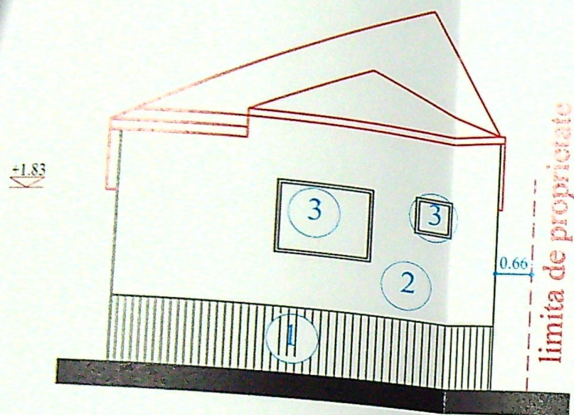
FATADA EST
