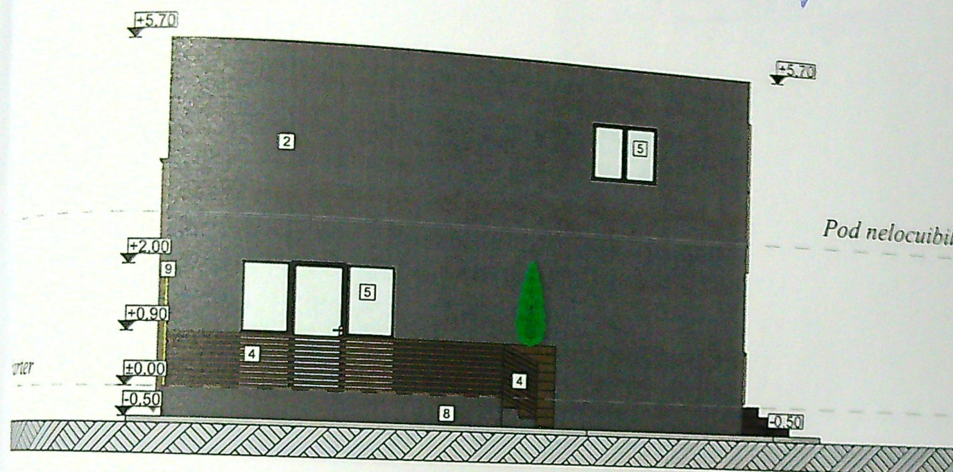
Fațadă lateral stânga -Est scara 1:100
