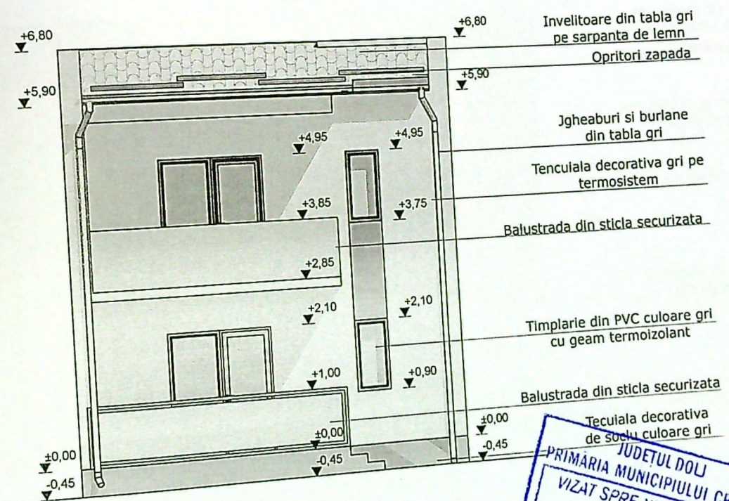
FATADA EST SCARA1:100
