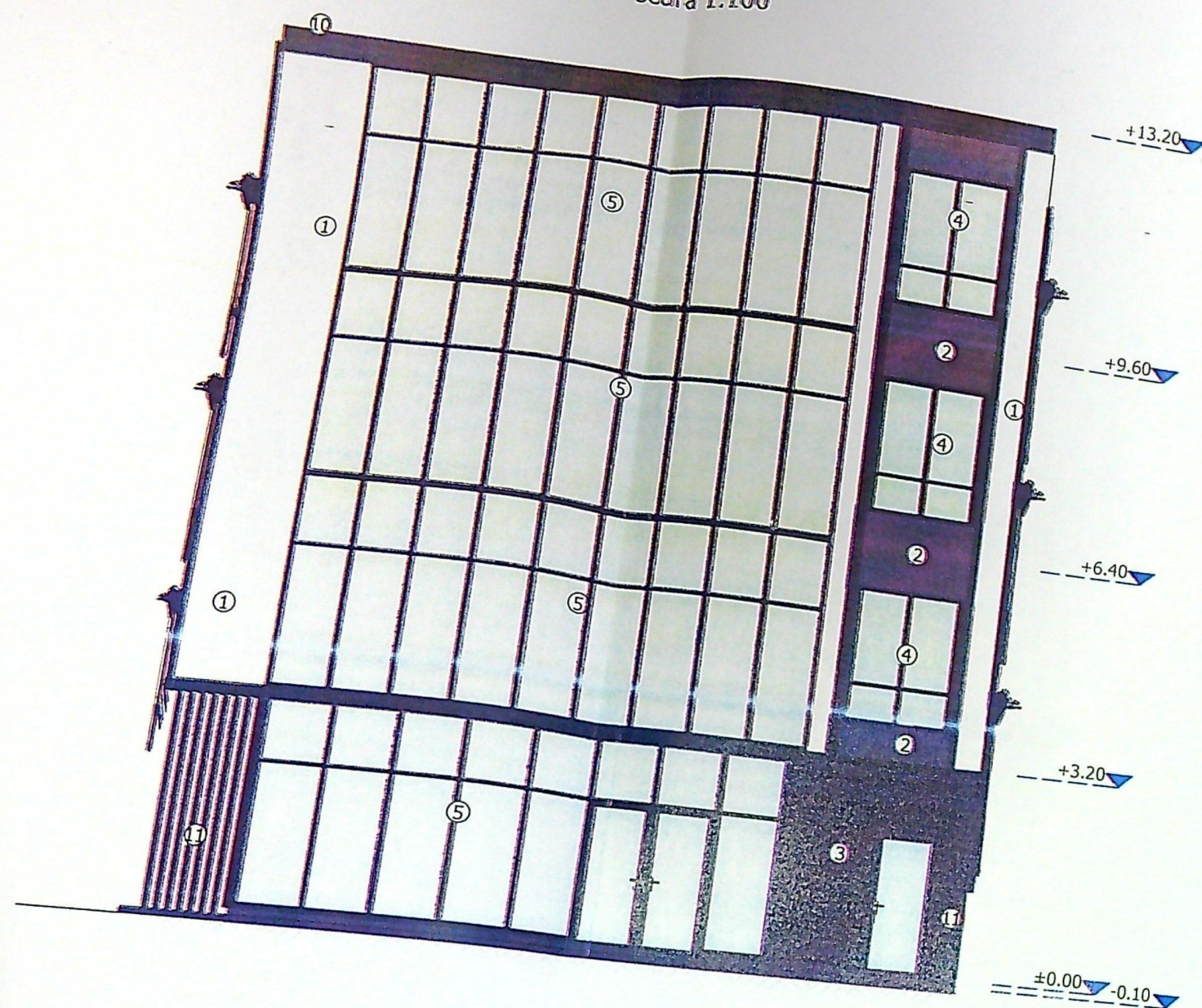
FATADA NORD scara 1:100
