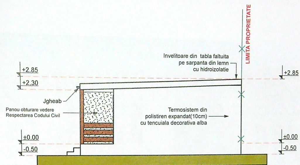
FATADA LATERALA DREAPTA Scara 1:100
