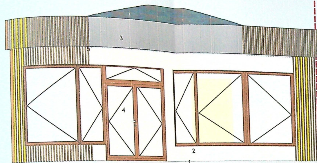
FAȚADĂ SUD-EST SC:1/50
