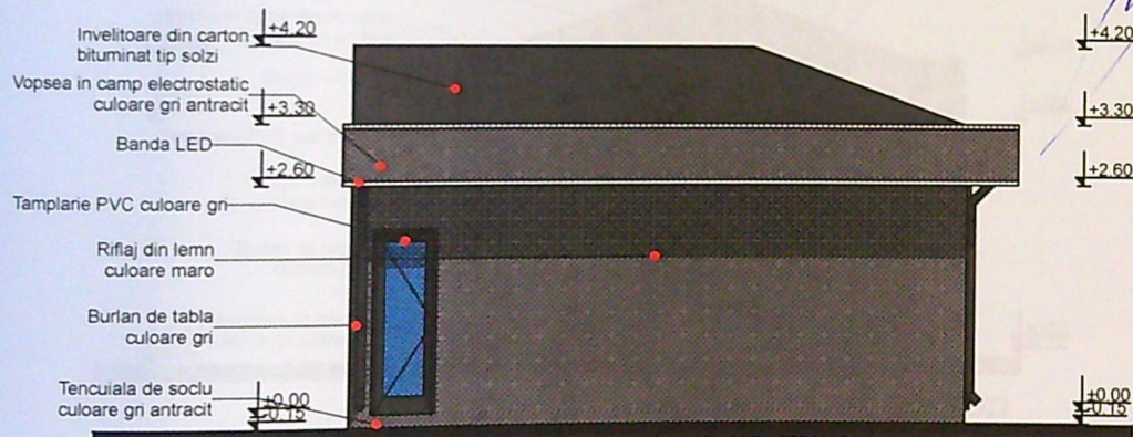
FATADA SECUNDARA VEST
