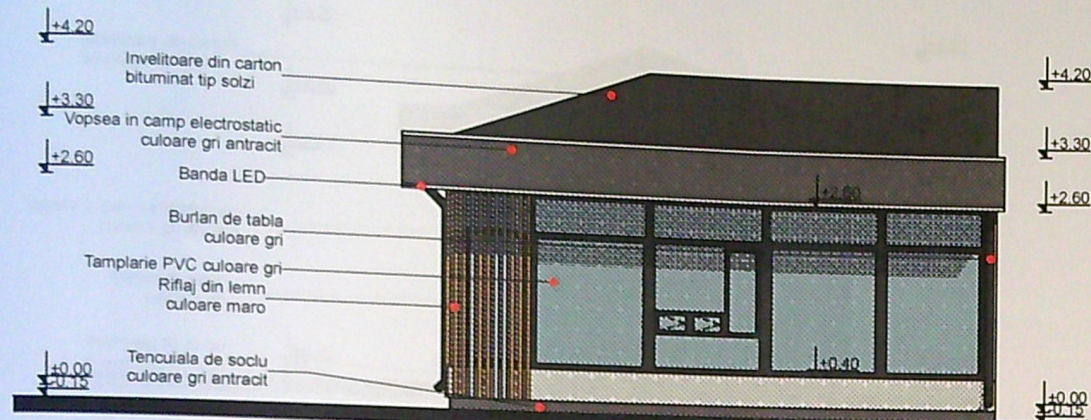
FATADA PRINCIPALA EST
