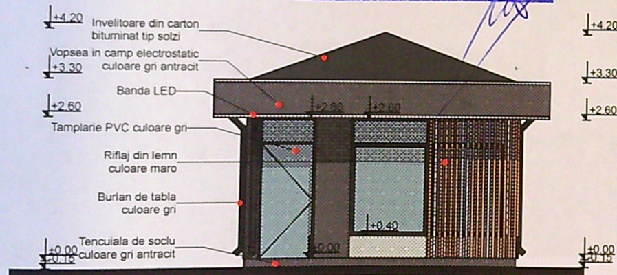
FATADA LATERALA SUD
