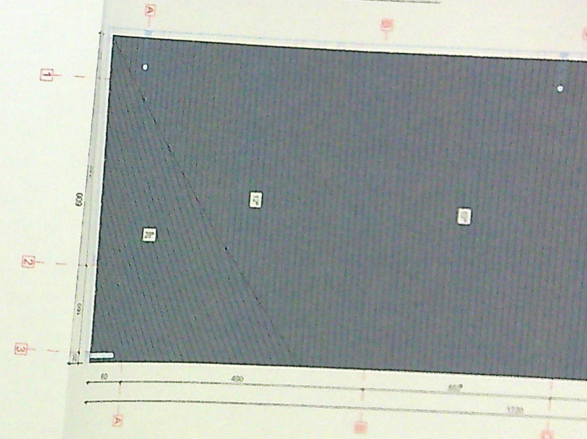
PLAN INVELITOARE scara : 1 / 100
