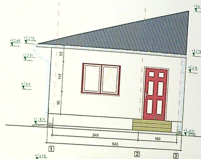
FATADA SUD - VEST scara : 1 / 100
