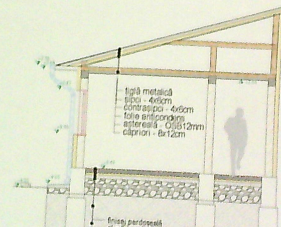
SECTIUNE A-A scara : 1 / 100
