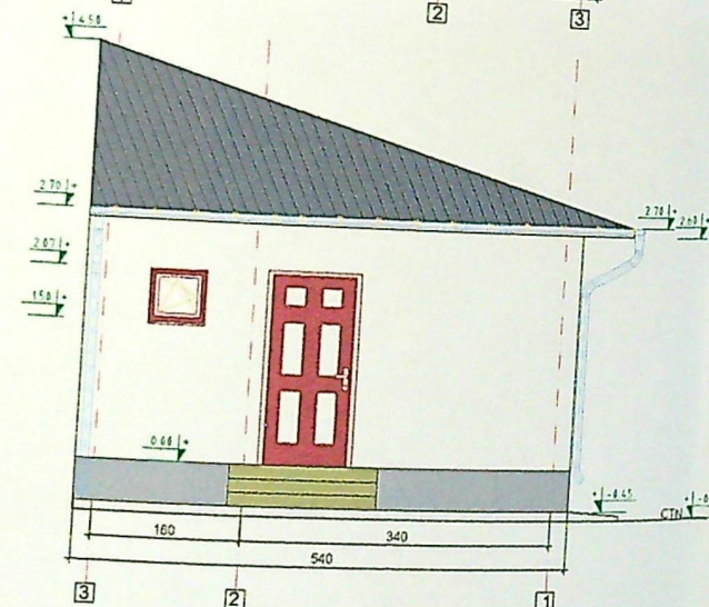
FATADA NORD - EST scara : 1 / 100
