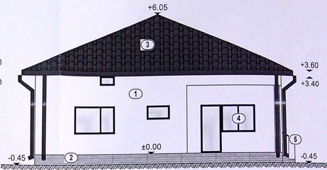
FATADA POSTERIOARA SC. 1:100
