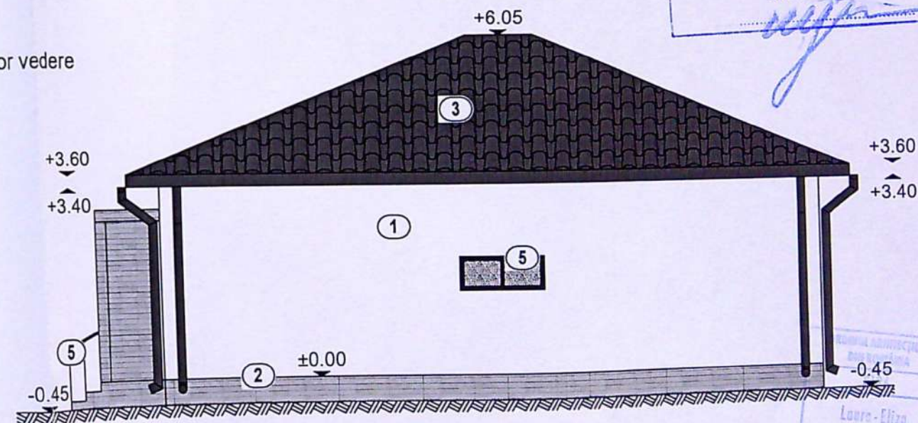
FATADA LAT.-DREAPTA SC. 1:100
