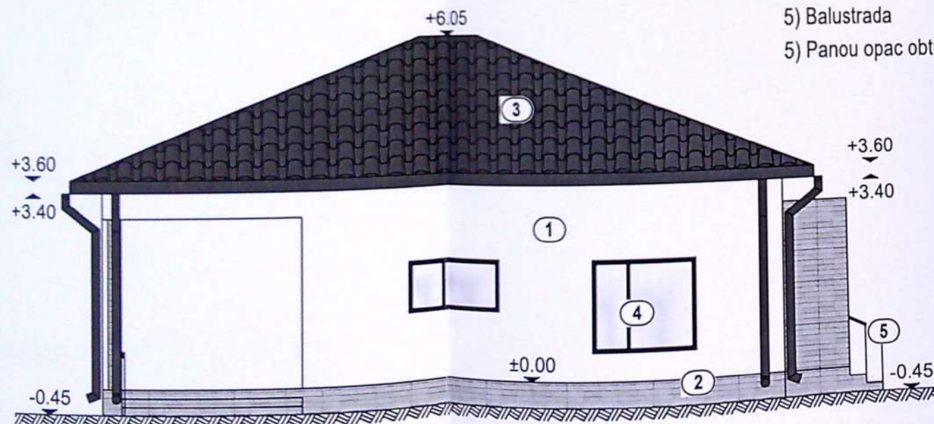
FATADA LAT.-STANGA SC. 1:100
