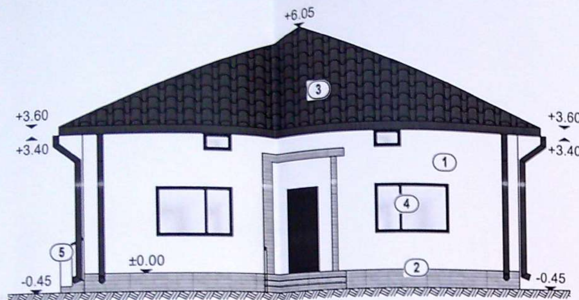
FATADA PRINCIPALA SC. 1:100
