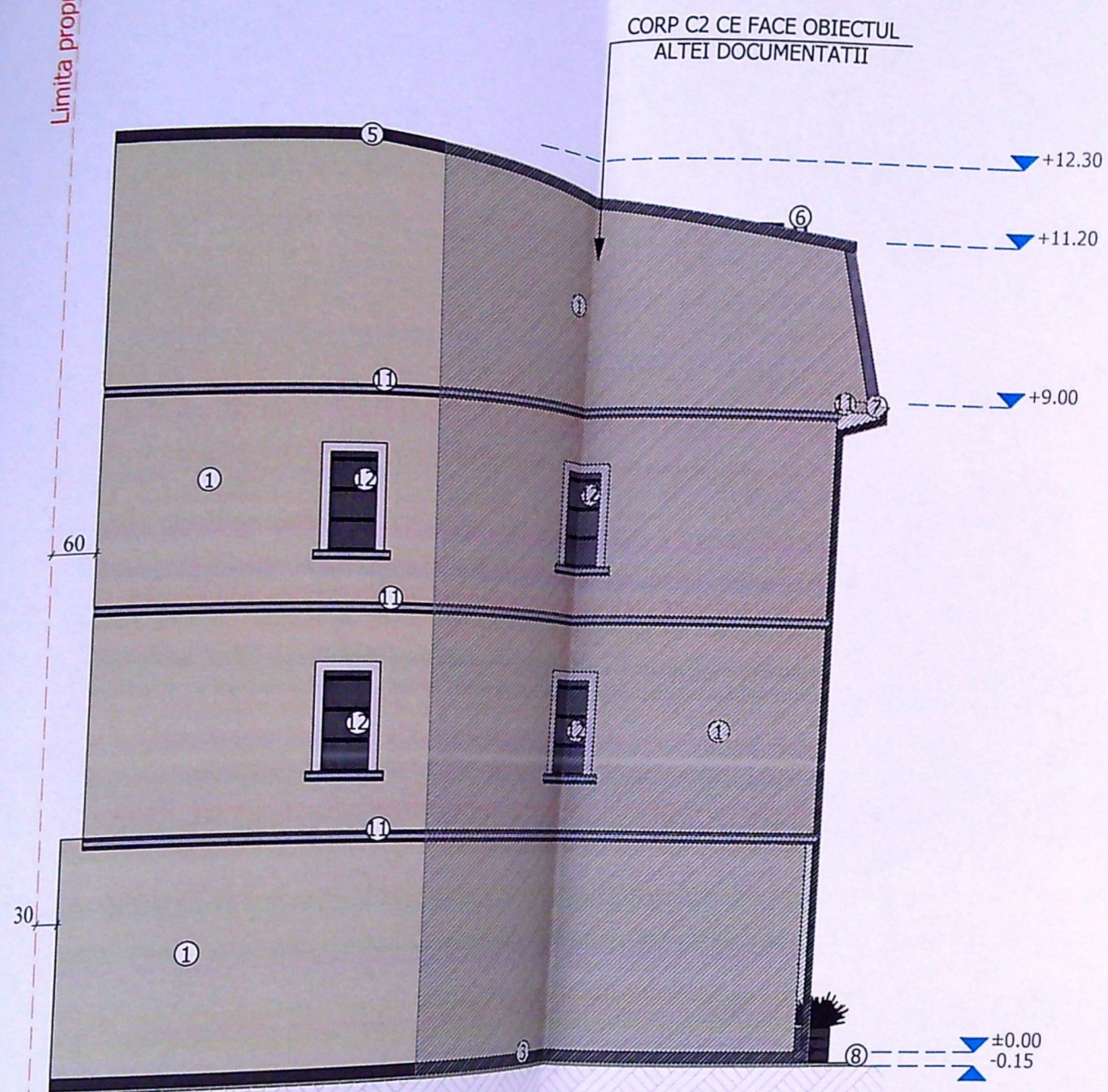
FATADA VEST PROPUS scara 1:100
