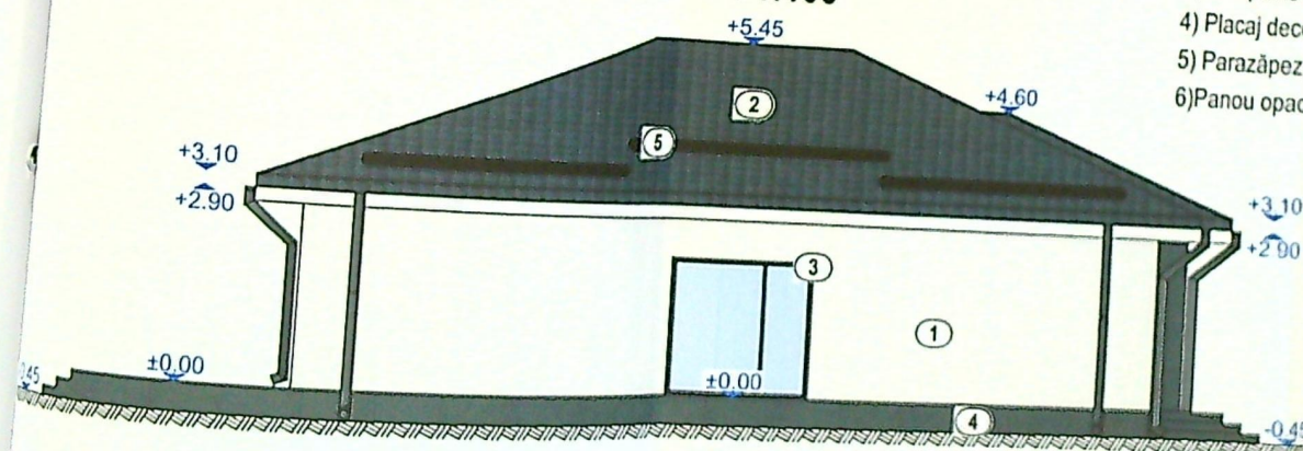
FAȚADA LAT.-STÂNGA SC. 1:100
