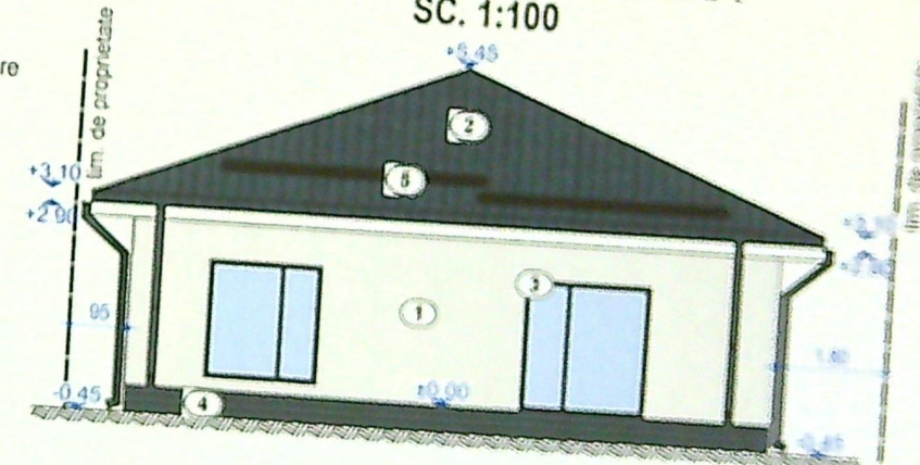
FATADA POSTERIOARĂ SC. 1:100
