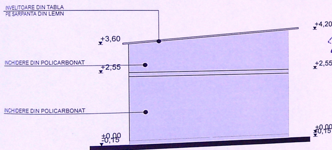
FATADA VEST SCARA 1:100
