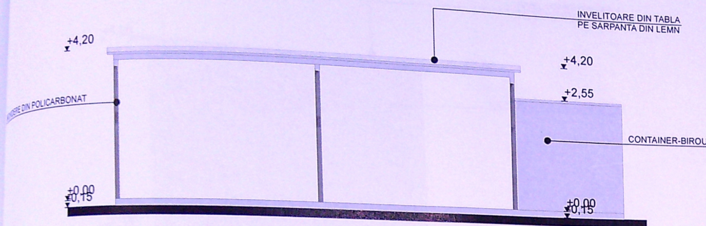
FATADA SUD SCARA 1:100
