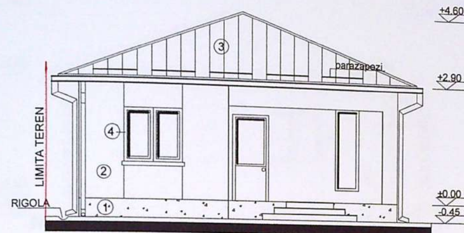
FATADA PRINCIPALA - NORD-VEST
