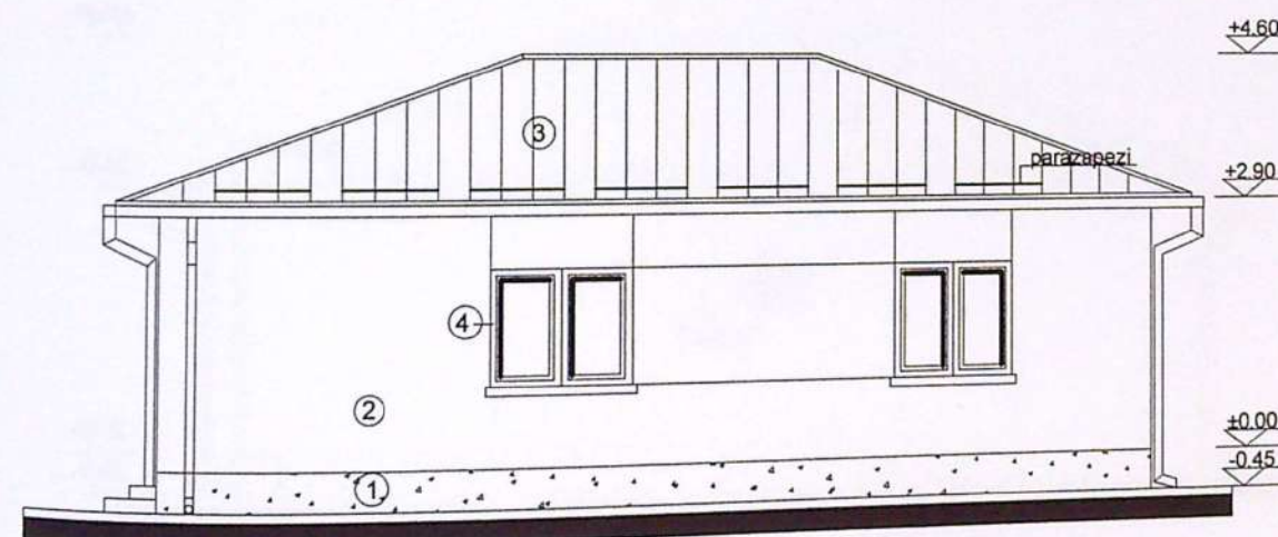
FATADA LATERALA DREAPTA - SUD-VEST
