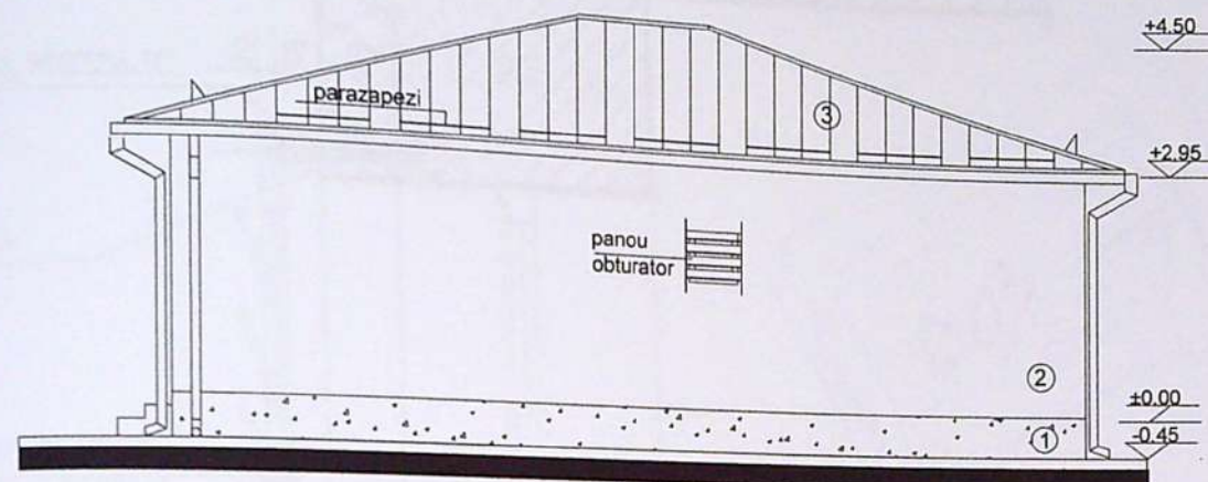
FATADA SECUNDARA - NORD-EST
