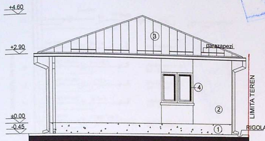
FATADA SECUNDARA - SUD-EST
