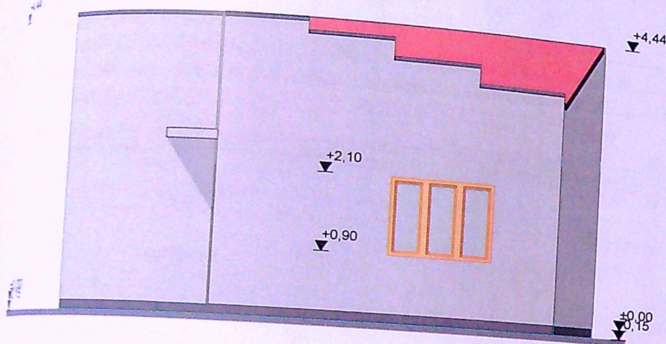
FATADA EST SCARA1:100
