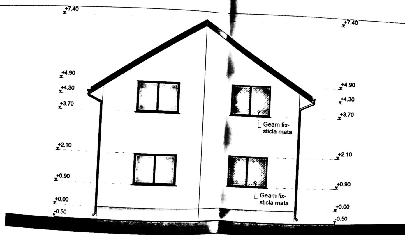
FATADA POSTERIOARA
