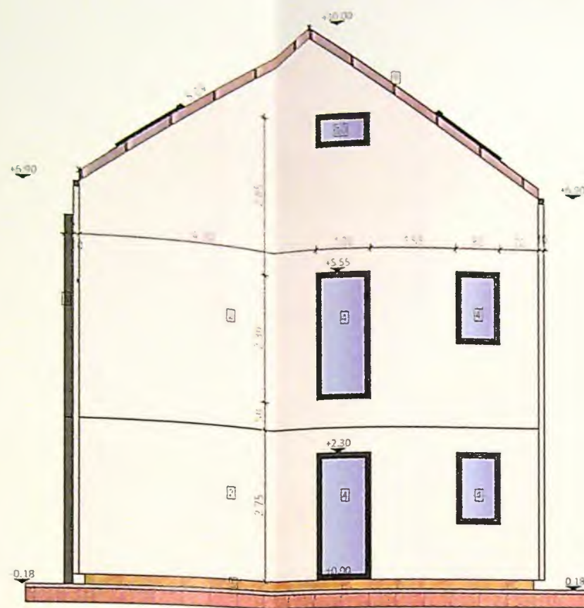
FATADA NORD-EST
