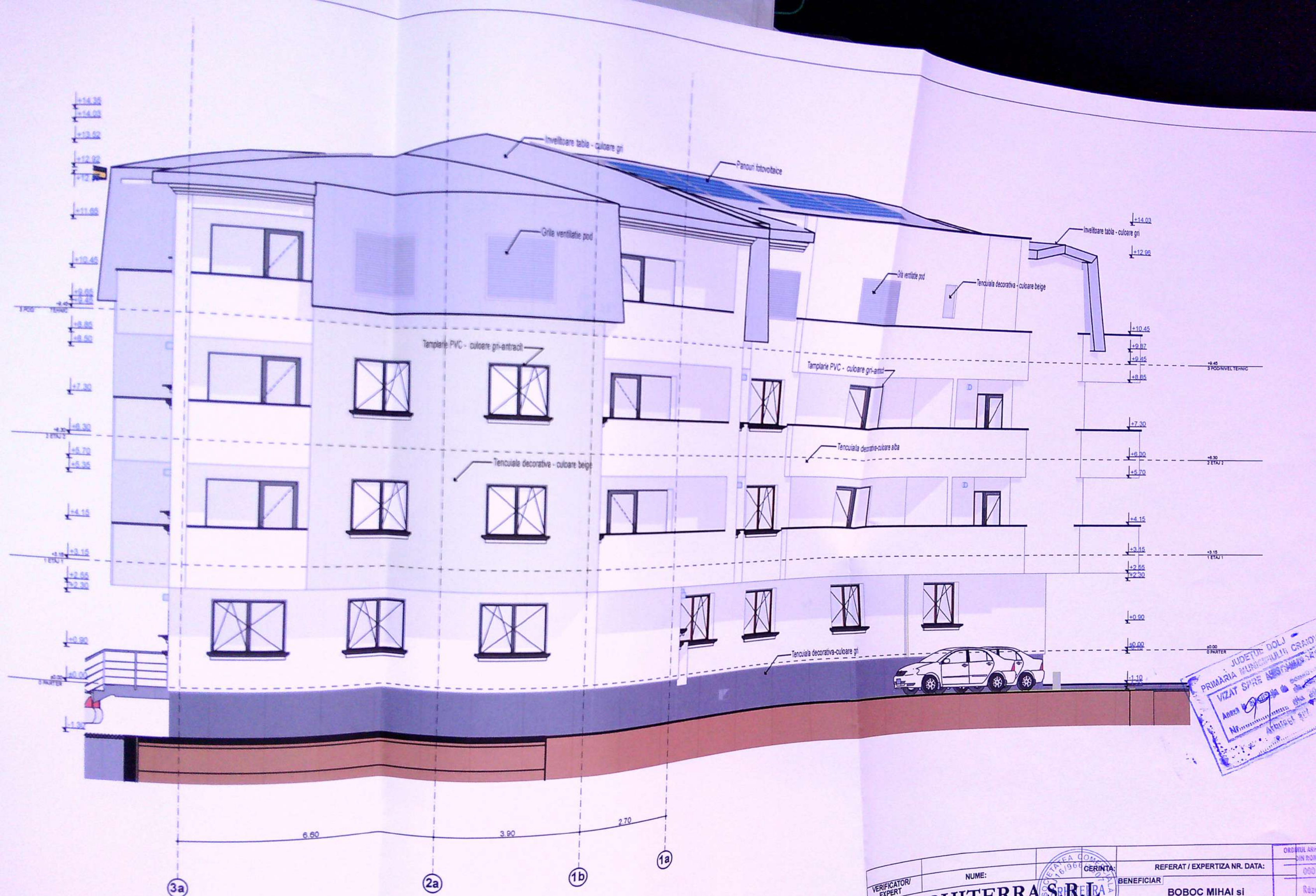
FATADA NORD - VEST - Corp C1
