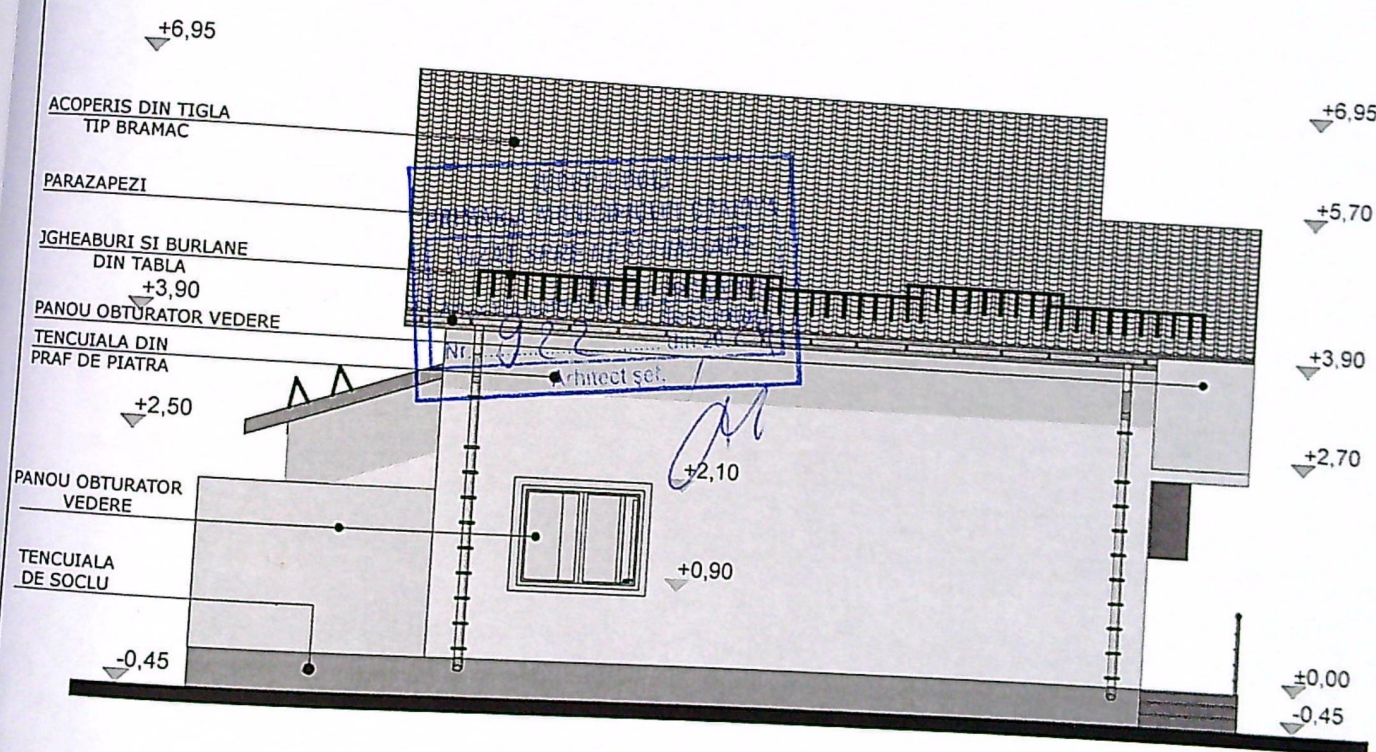
FATADA VEST SCARA 1:100
