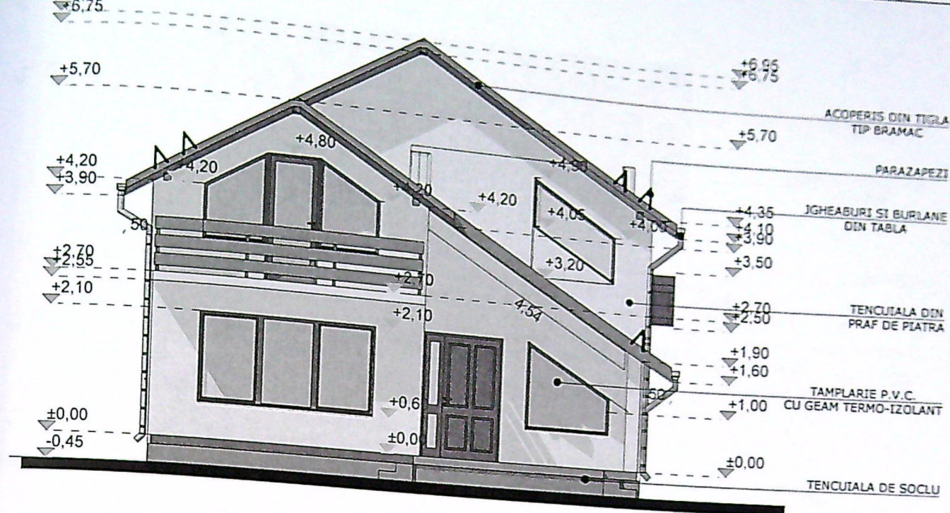
FATADA SUD SCARA 1:100
