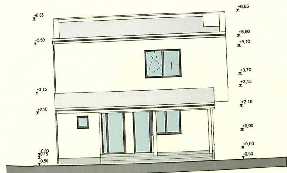
FATADA POSTERIOARA
