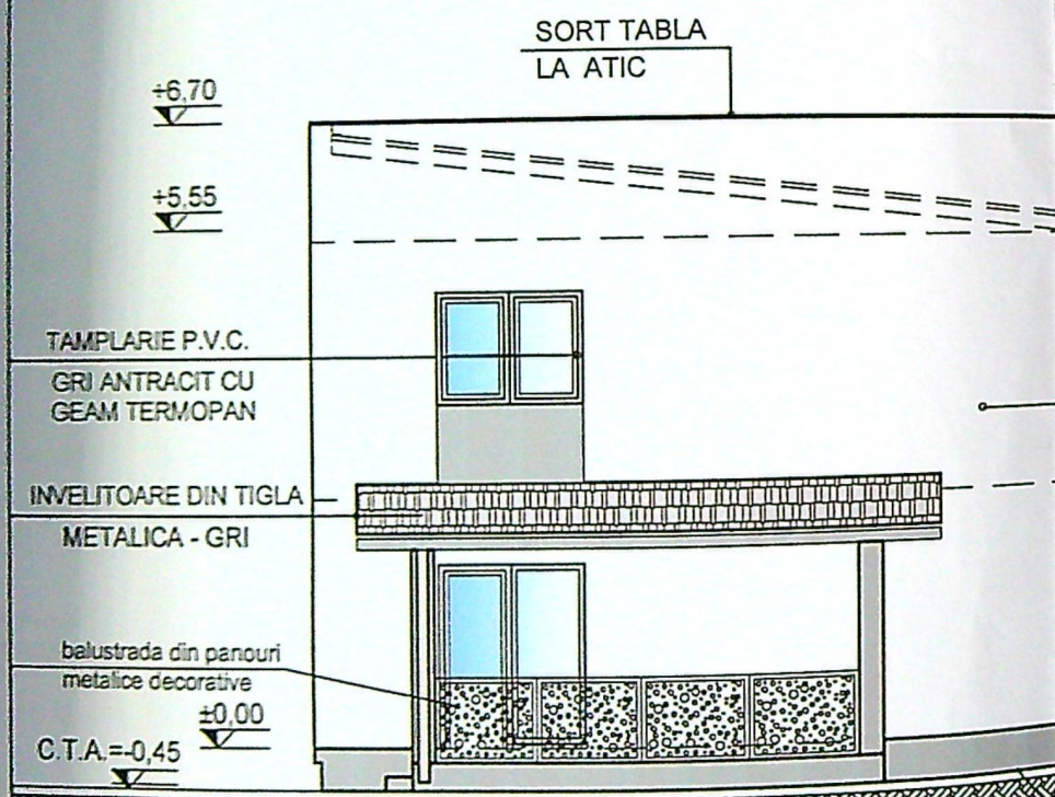
FATADA PRINCIPALA - (NORD-EST) scara 1 : 100
