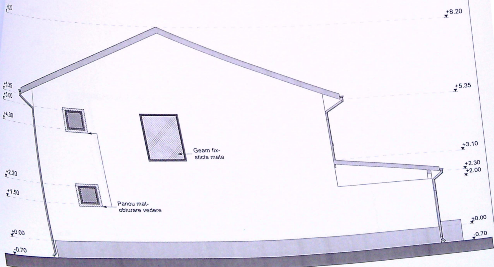
FATADA POSTERIOARA
