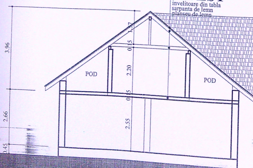
SECTIUNEA A-A
