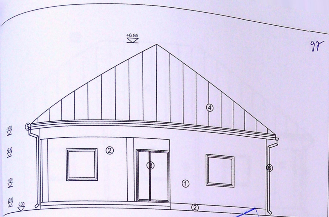
FATADA SUD - SC. 1: 100
