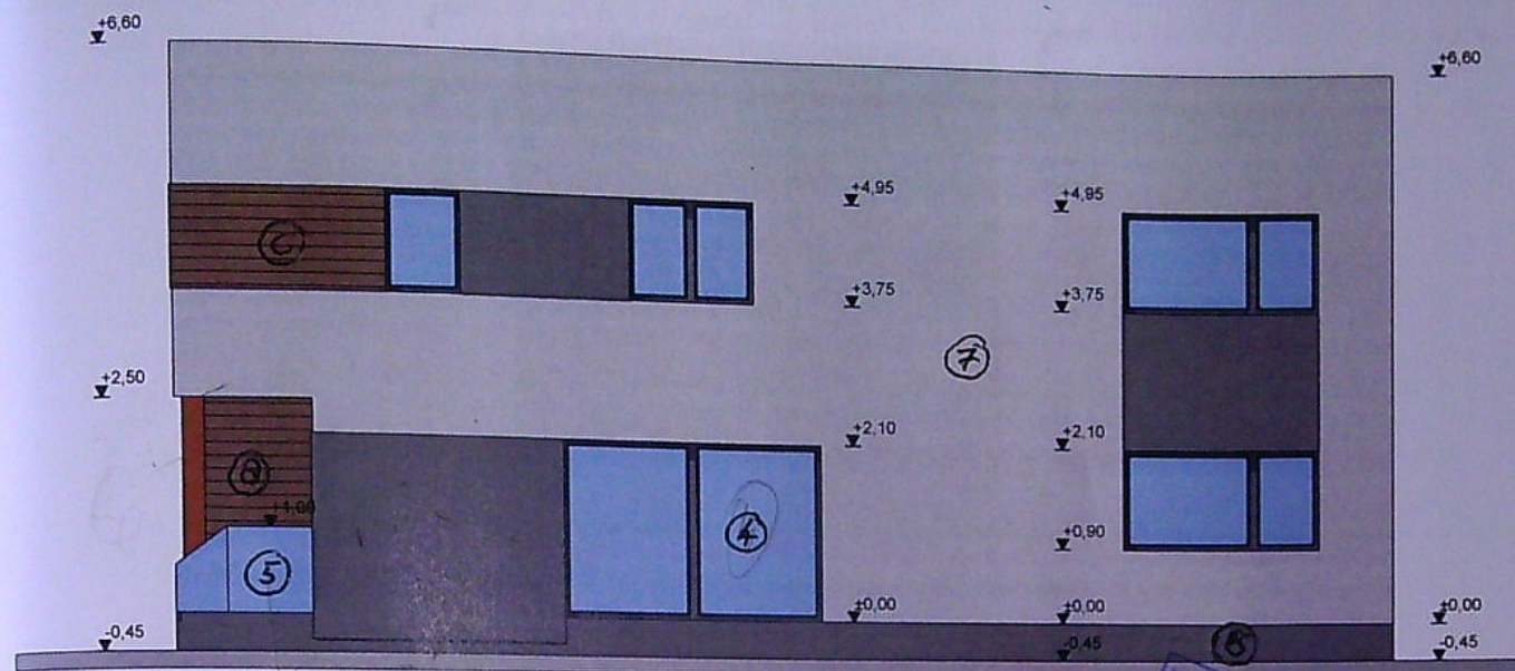
FATADA SUD SCARA1:100
