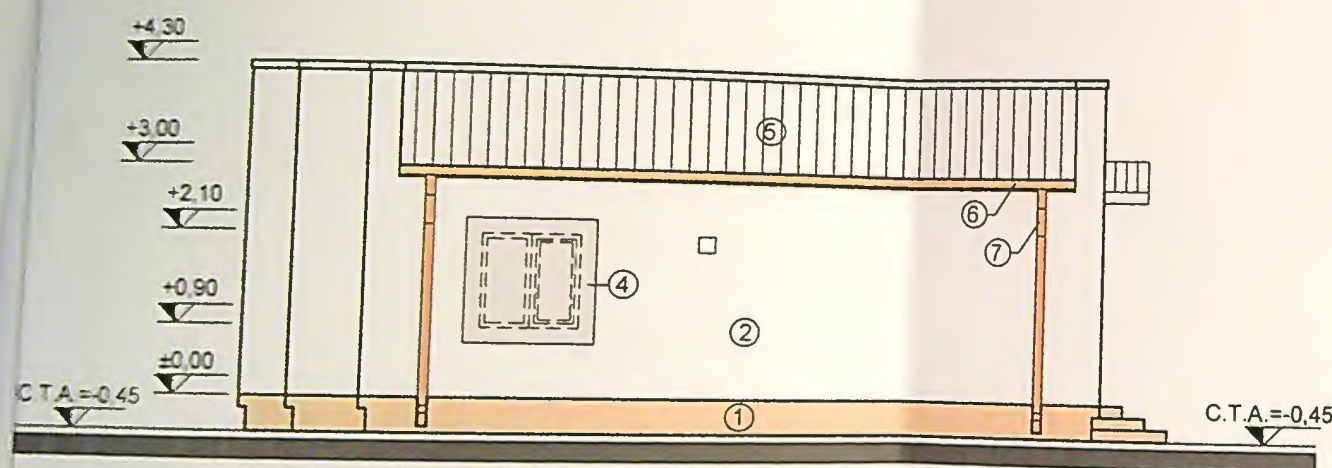
FATADA SECUNDARA (SUD - EST)
