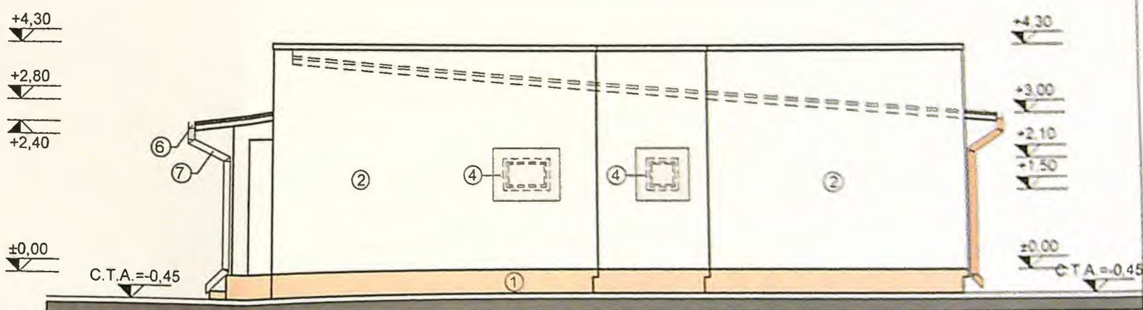
FATADA LATERALA DREAPTA (SUD - VEST)
