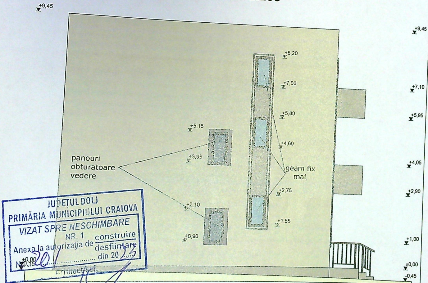
FATADA VEST SCARA 1:100
