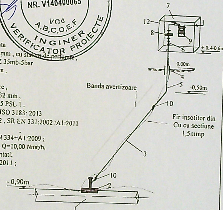
SCHEMA IZOMETRICA RACORD GAZE NATURALE R.P.
