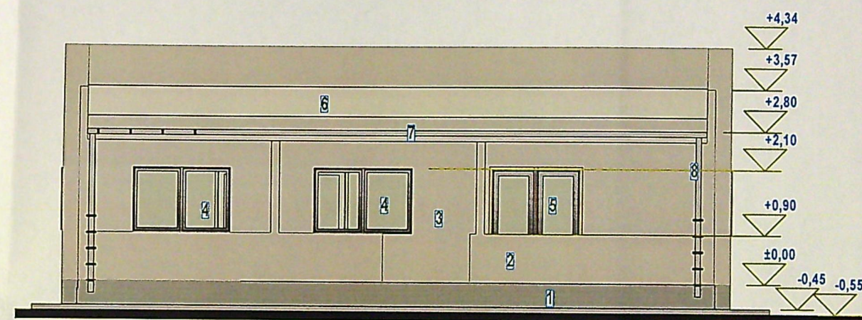
FATADA SECUNDARA (DE NORD-VEST) Finisaje: 1-soclu impermeabil gr; 2-parapet de protecție terasă; 3-vopsea lavabila alba; 4-fereșre PVC antracit; 5-usa PVC antracit cu geam securizat; 6-invelitoare din panouri isopan; 7-igheab; 8-burlan
