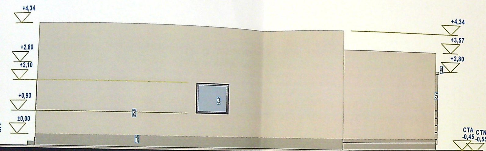
FATADA LATERALA DREAPTA (DE NORD-EST) Finisaje: 1-soclu impermeabil gr; 2-vopsea lavabila alba; 3-fereastră fixa opacă; 4-igheab; 5-burlan
