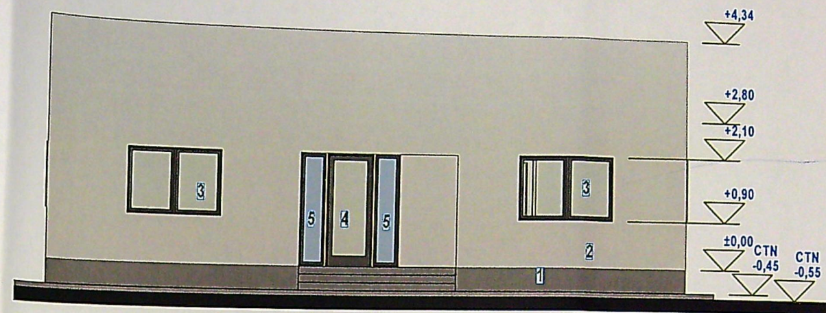
FATADA PRINCIPALA (de sud-est) Finisaje: 1-soclu impermeabil gr; 2-vopsea lavabila alba; 3-fereastră PVC antracit; 4-usa metalica antracit; 5-fereșre fixe cu geam securizat
