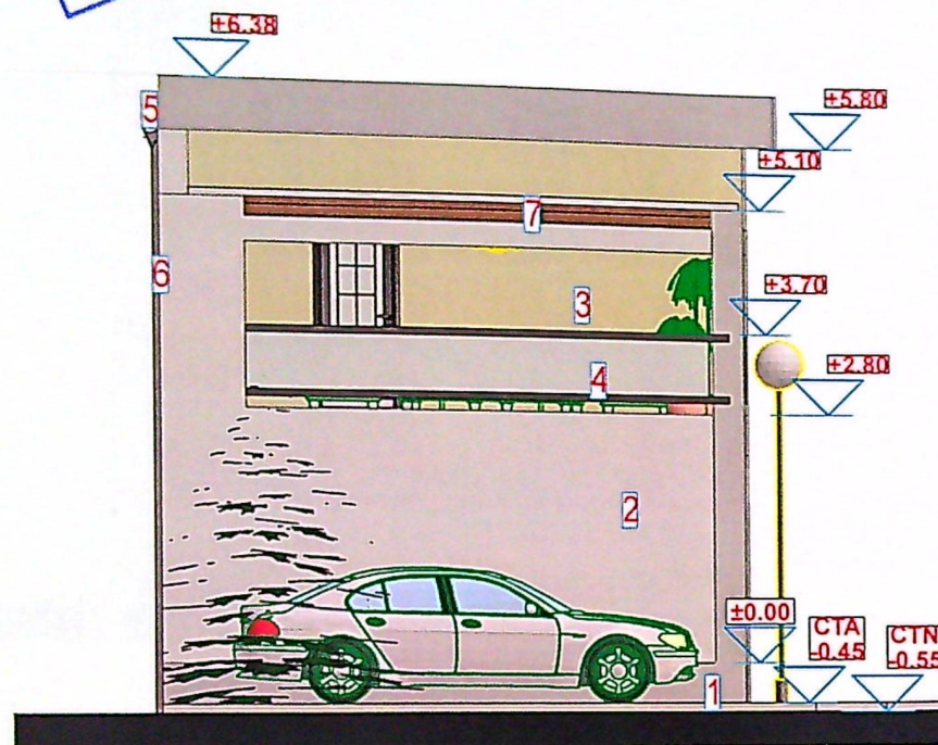
FATADA DE SUD LA C4
