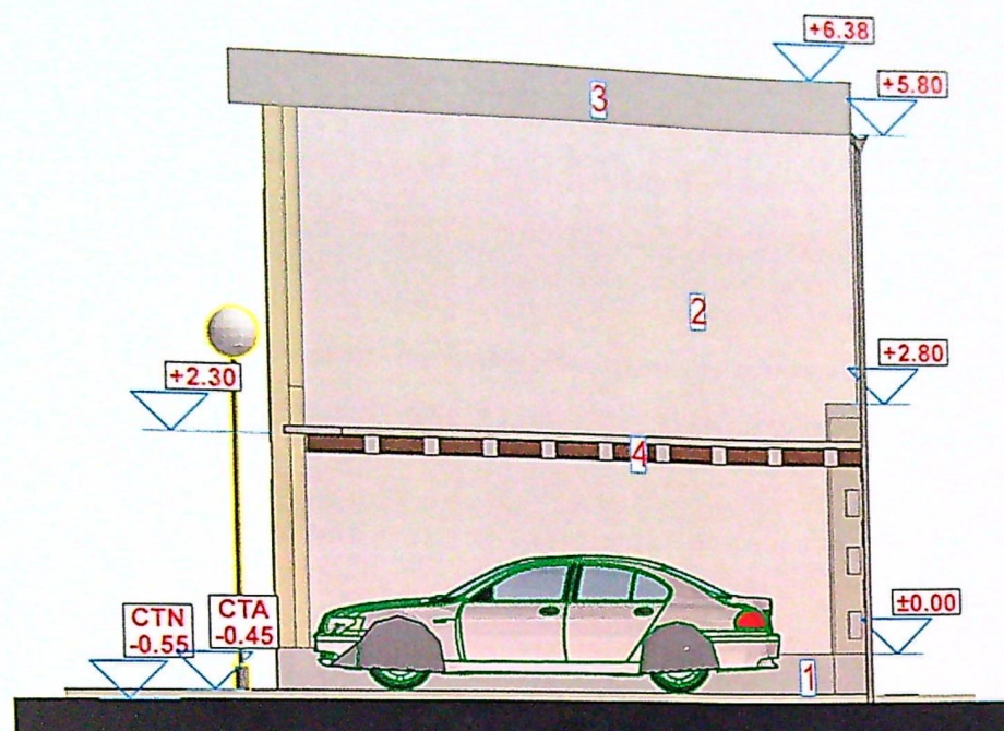
FATADA DE NORD LA C5
