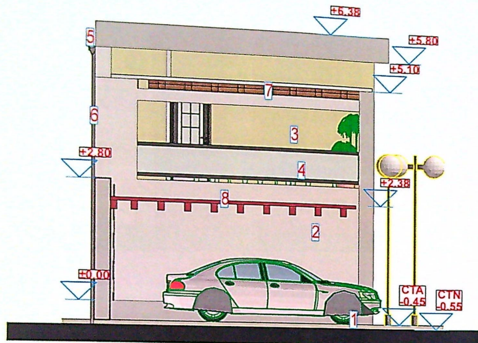
FATADA DE SUD LA C6
