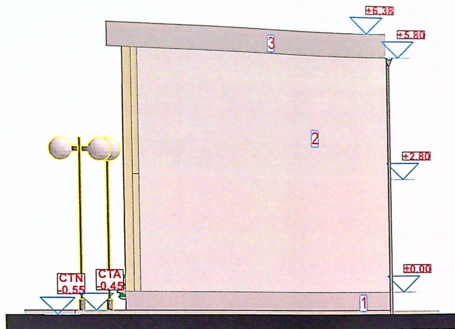
FATADA DE NORD LA C7
