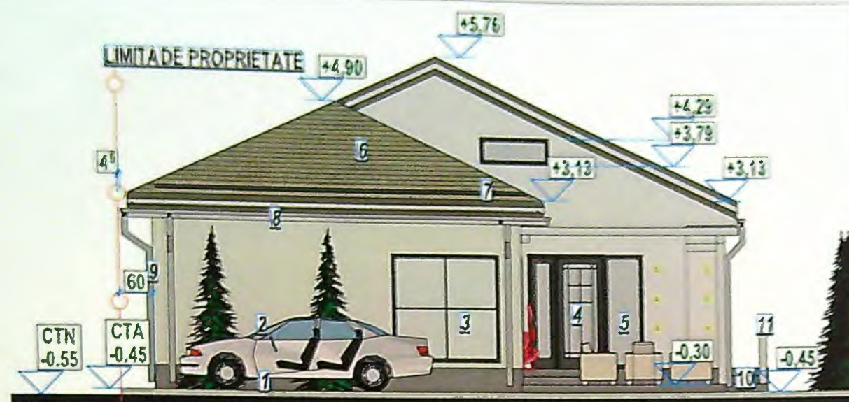
FATADA PRINCIPALA (DE SUD-EST)
