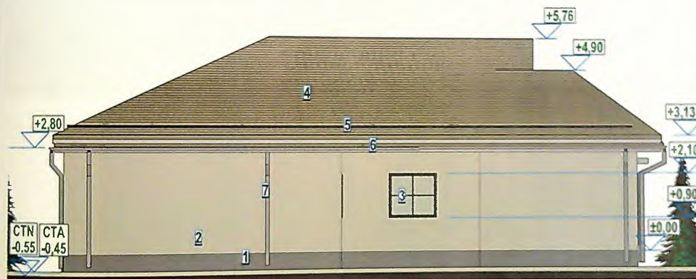
FATADALATERALA DREAPTA/DE SUD-VEST
