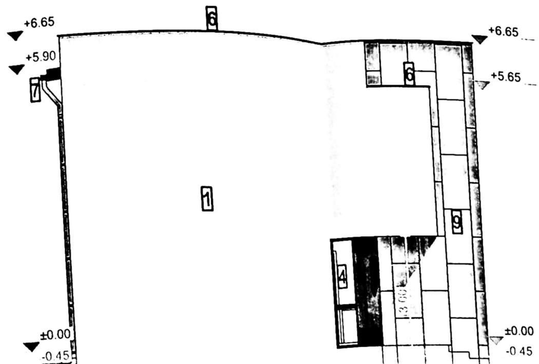
FATADA NORD
