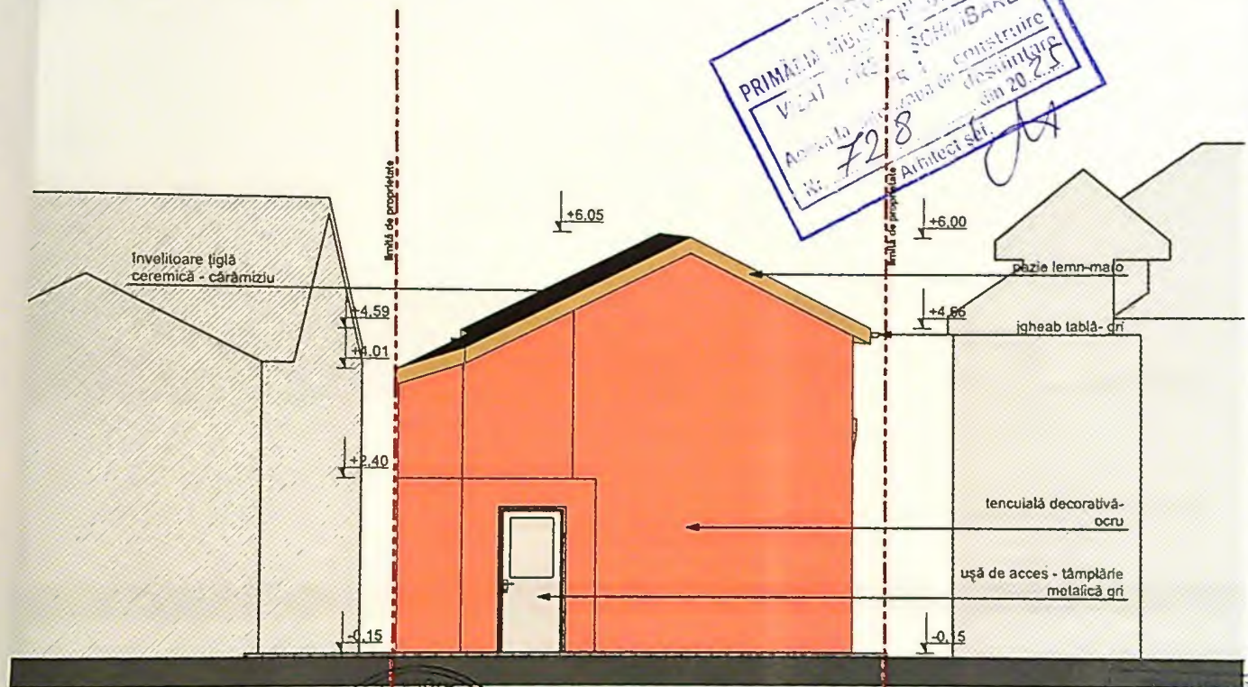
FAȚADĂ EST
