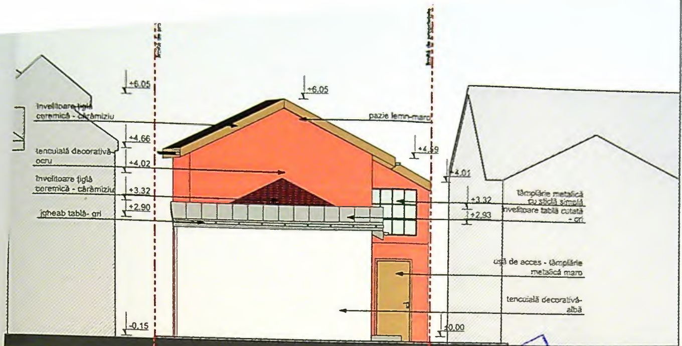
FAȚADĂ VEST
