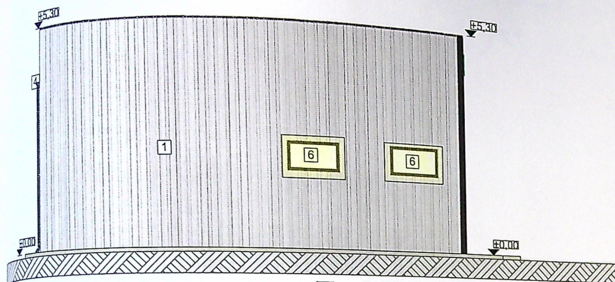
Fațadă lateral stânga -Est scara 1:100
