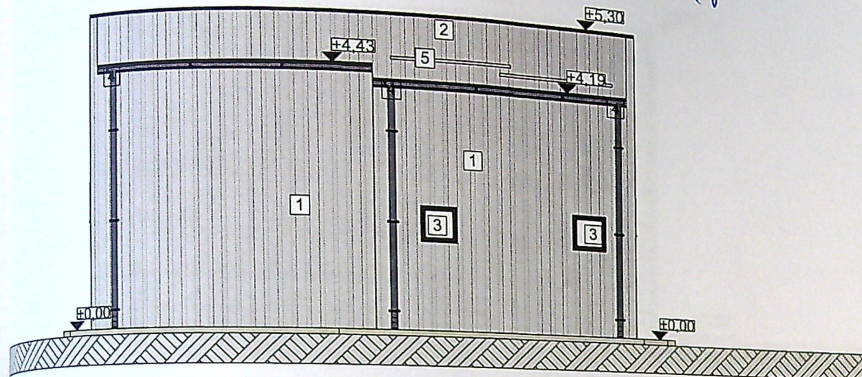
Fațadă posterioară -Sud scara 1:100
