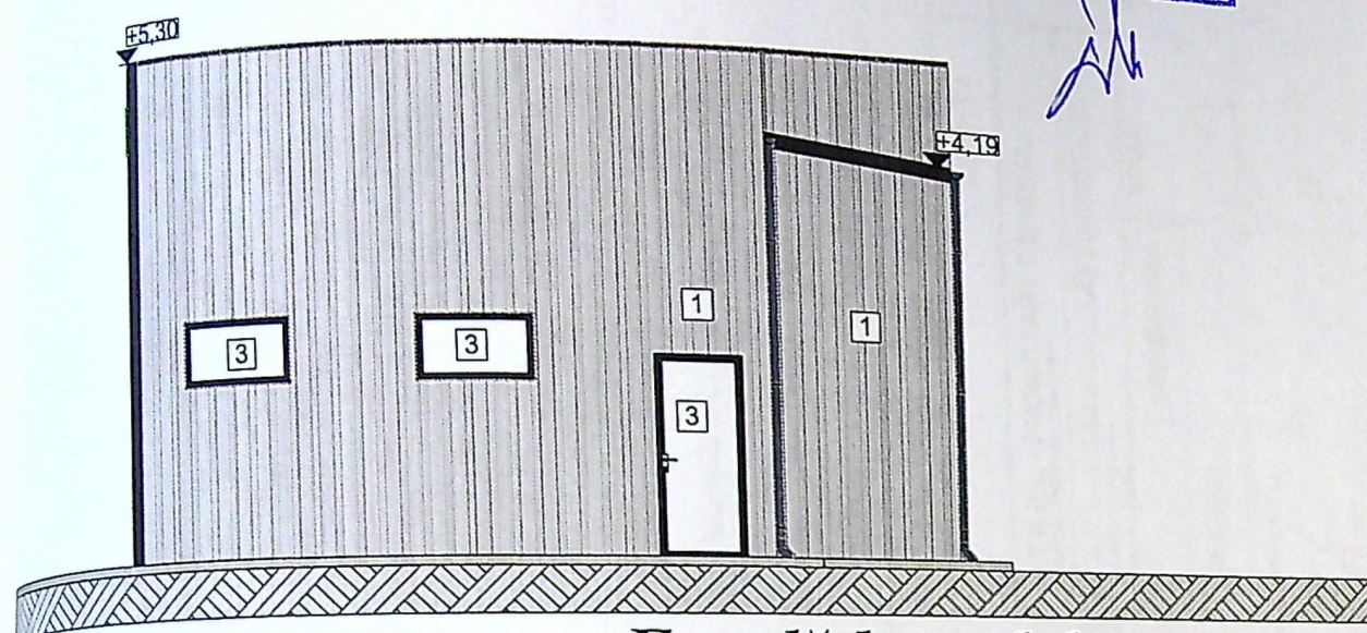
Fațadă lateral dreapta - Vest scara 1:100
