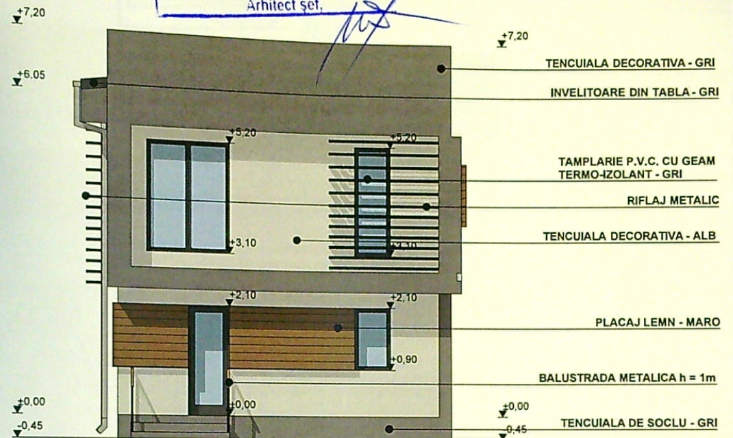
FATADA EST
