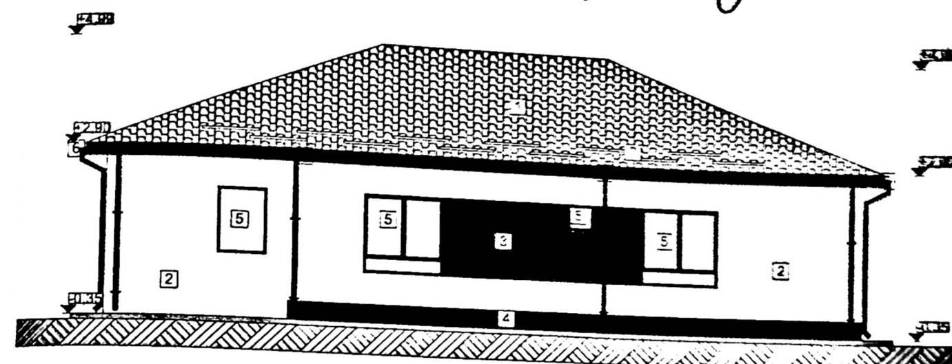
Fațadă posterioară locuință - Nord scara 1:100
