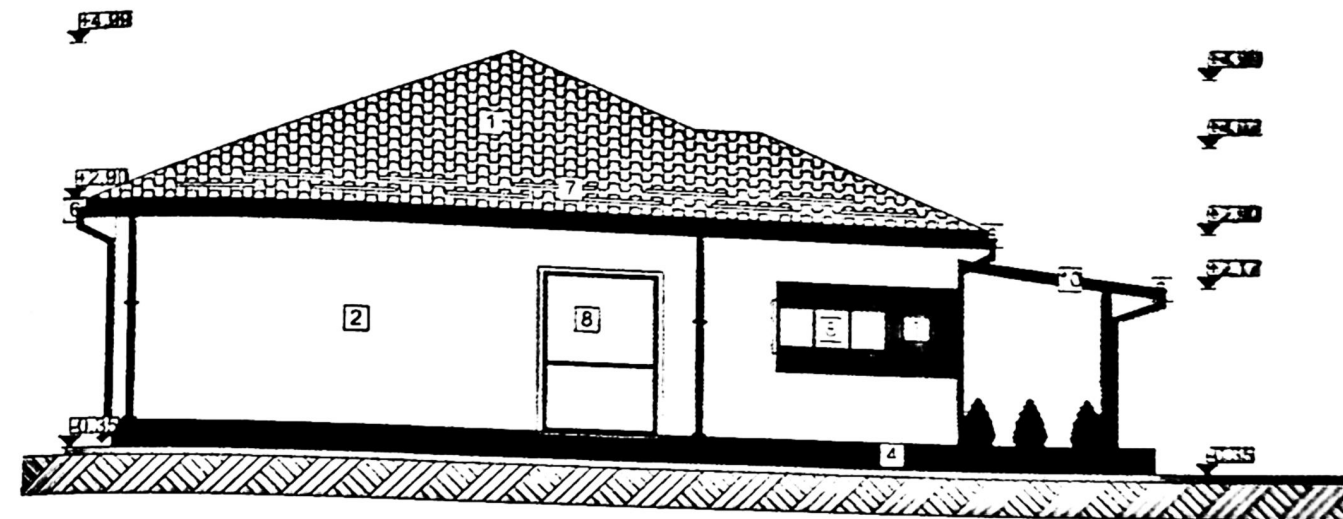
Fațadă lateral stânga -vest scara 1:100
