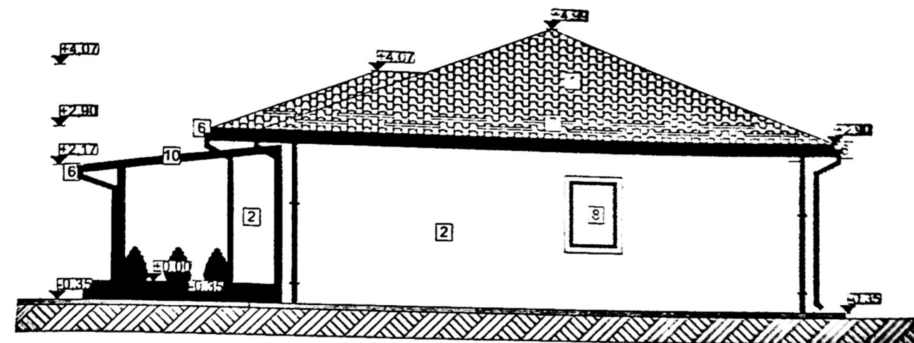
Fațadă lateral dreapta -est scara 1:100
