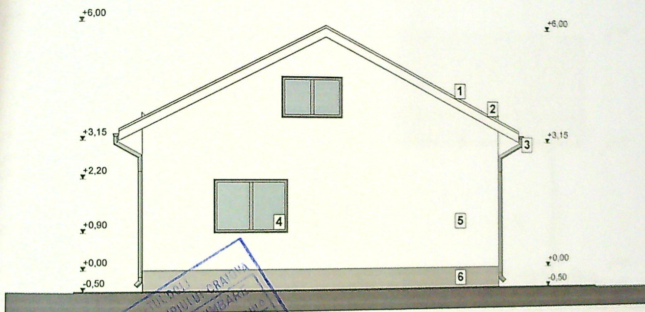
FATADA POSTERIOARA
