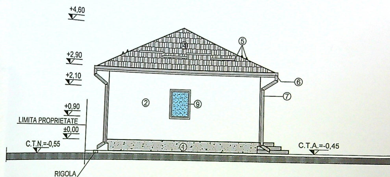
LOCUINTA C2 - FATADA LATERALA STANGA (SUD-VEST) scara 1 : 100
