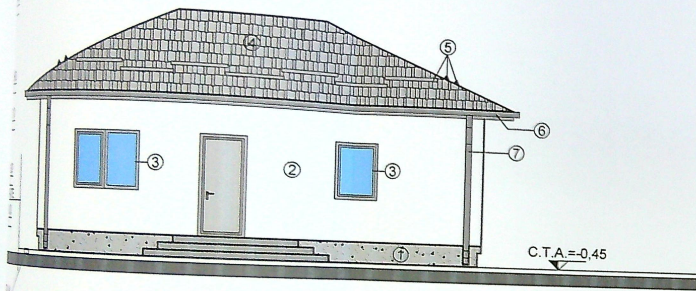
LOCUINTA C2 - FATADA PRINCIPALA (SUD-EST) scara 1 : 100
