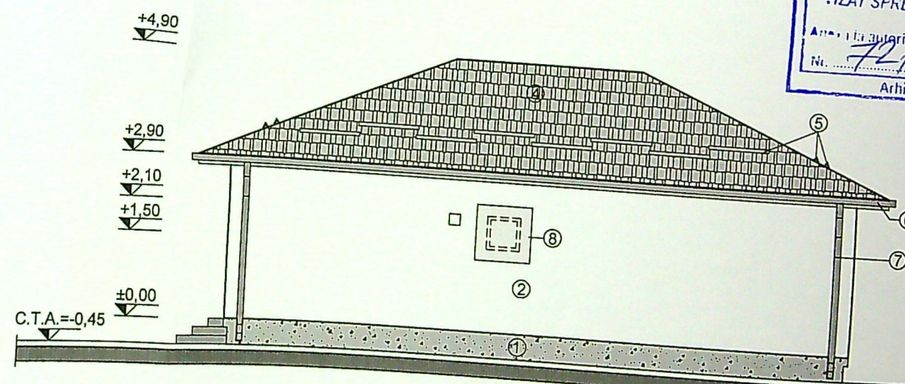
LOCUINTA C1 - FATADA LATERALA DREAPTA (NORD-EST) scara 1 : 100
