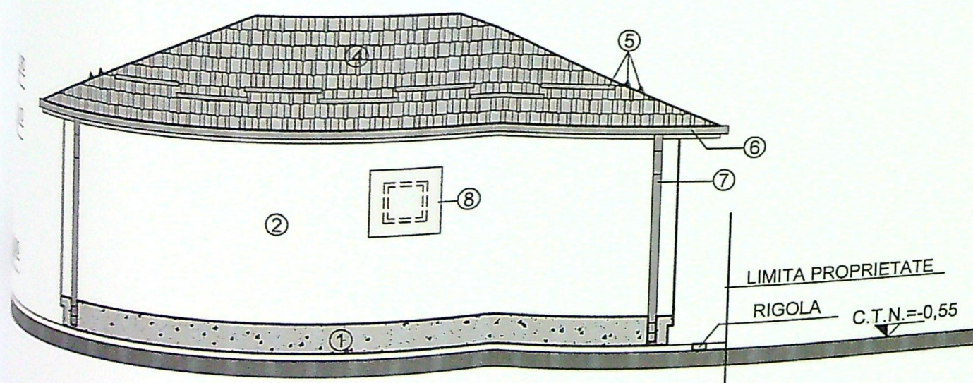
LOCUINTA C2 - FATADA SECUNDARA (NORD-VEST) scara 1 : 100
