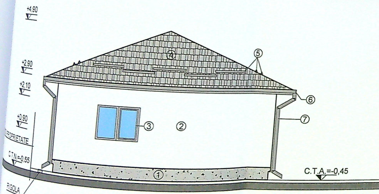
LOCUINTA C1 - FATADA SECUNDARA (NORD-VEST) scara 1 : 100
