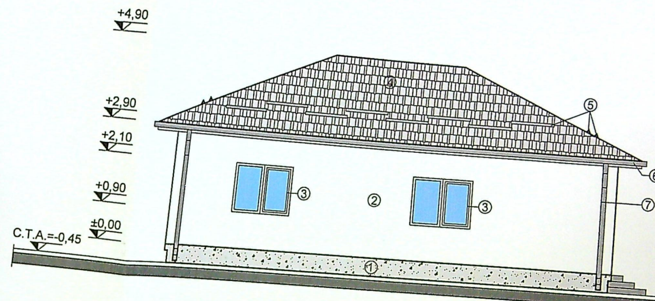
LOCUINTA C1 - FATADA LATERALA STANGA (SUD-VEST) scara 1 : 100
