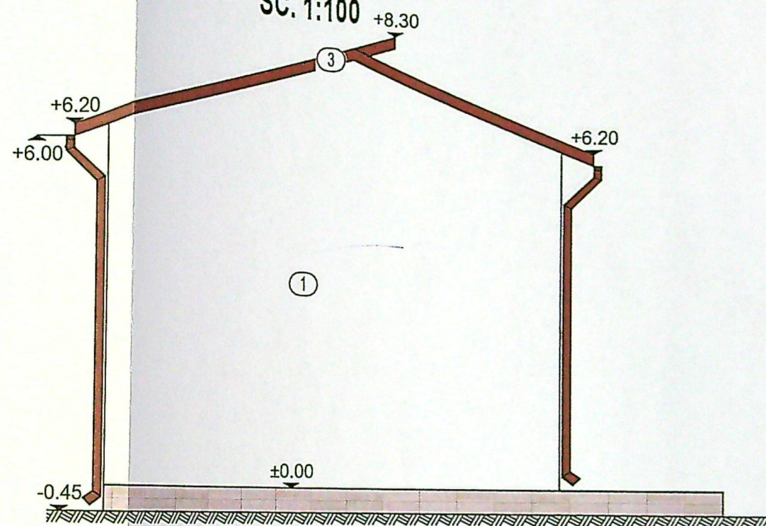
FAȚADA POSTERIOARĂ SC. 1:100
