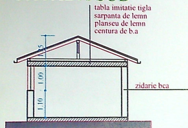
FATADA SUD
