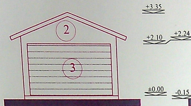
FATADA NORD
