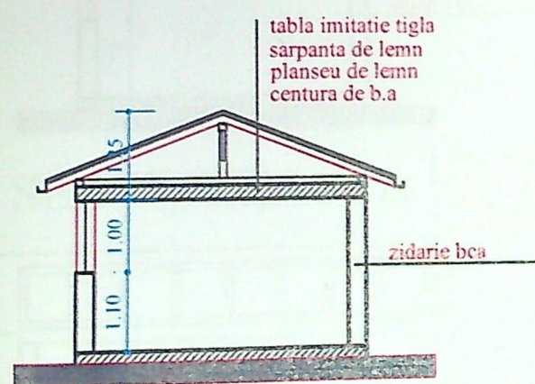
SECTIUNEA A-A
