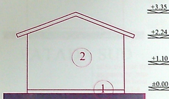
FATADA SUD
