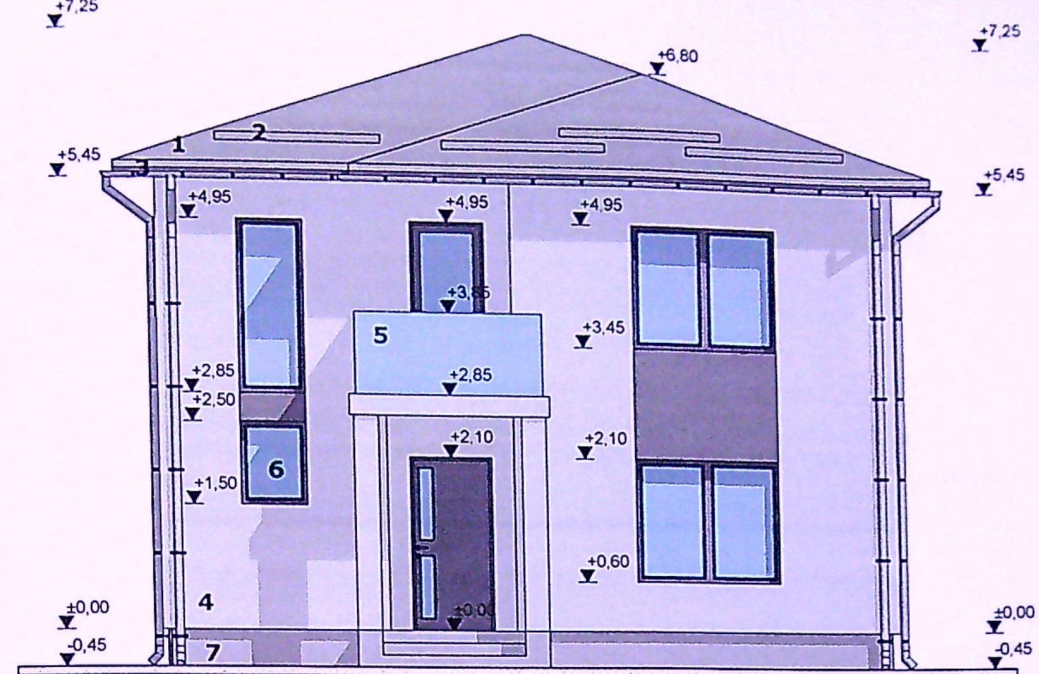
FATADA NORD SCARA 1:100
