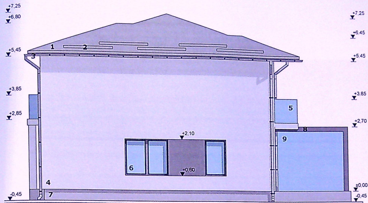
FATADA VEST SCARA 1:100
