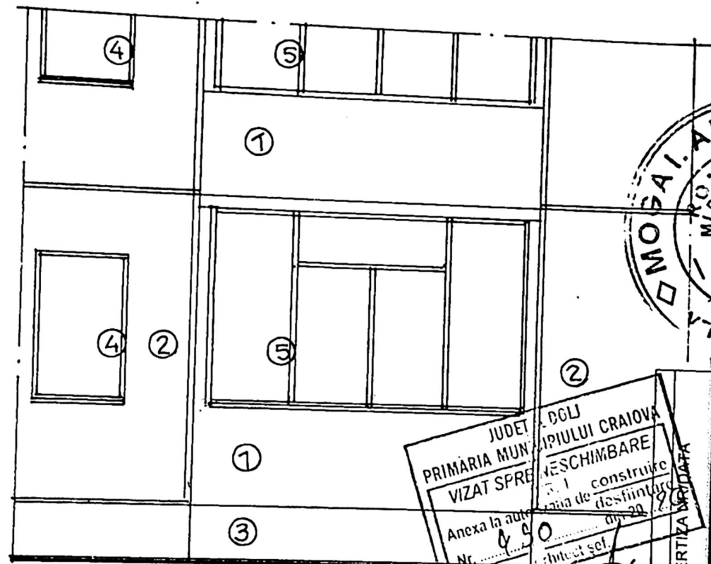
● ELEVATIE SUD
