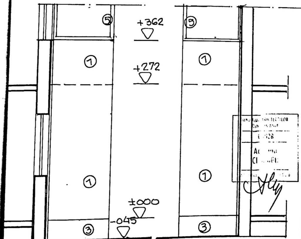
ELEVATIE EST
