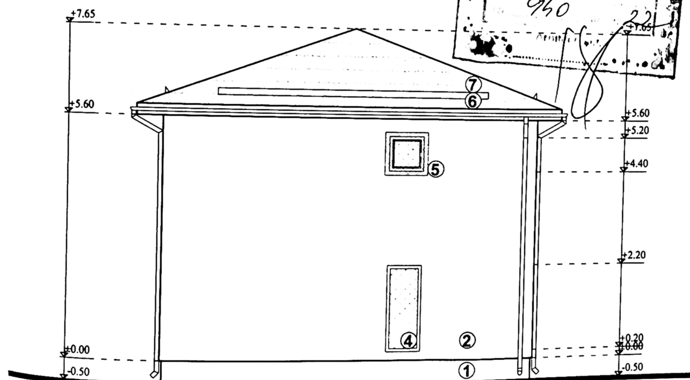
FATADA POSTERIOARA
