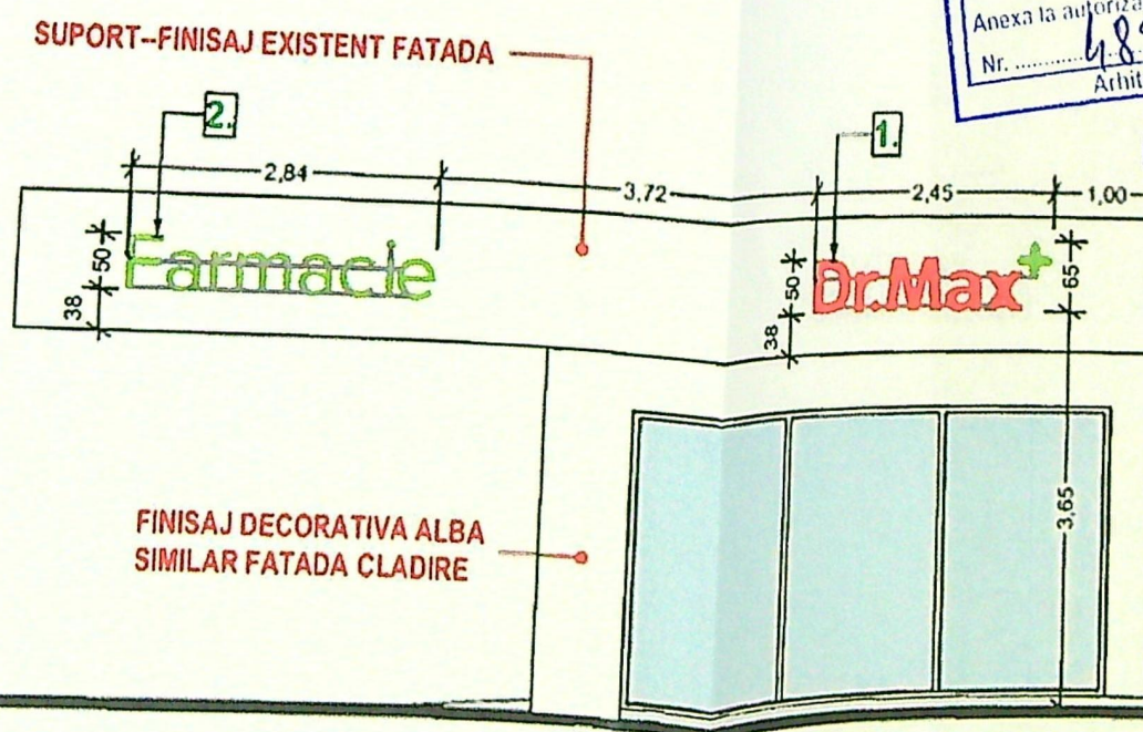
FATADA LATERALA PROPUSA
