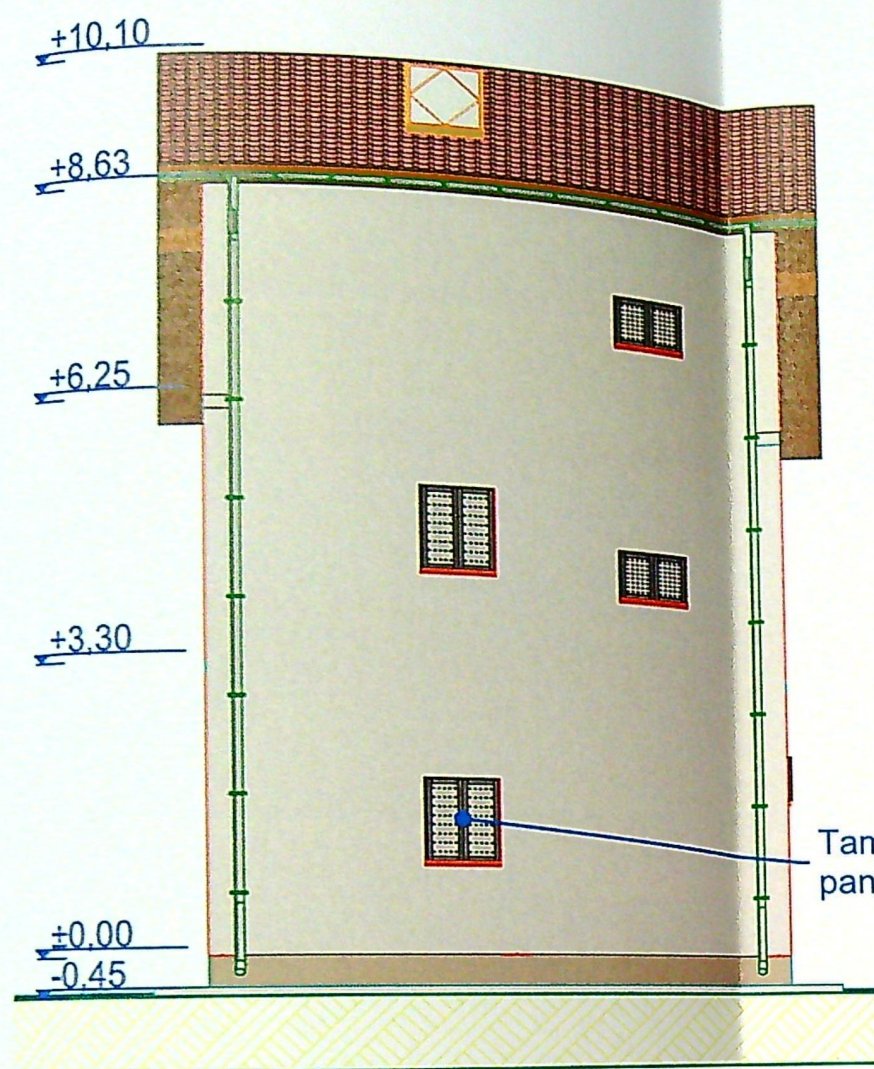
FATADA POSTERIOARA scara 1:100
