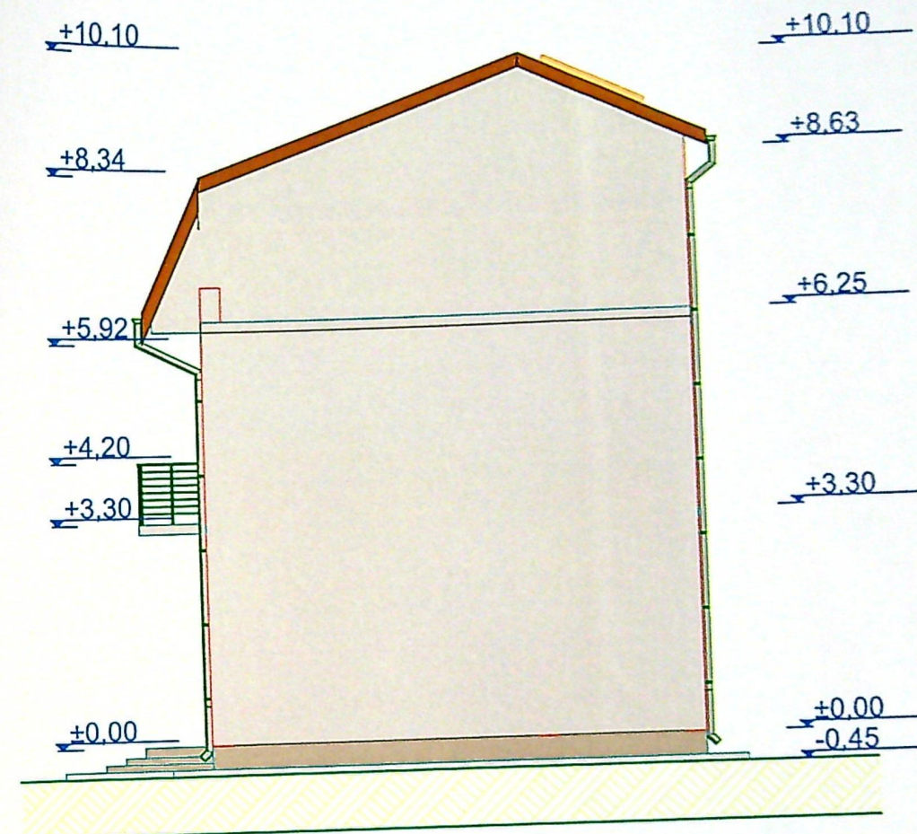
FATADA DREAPTA scara 1:100
